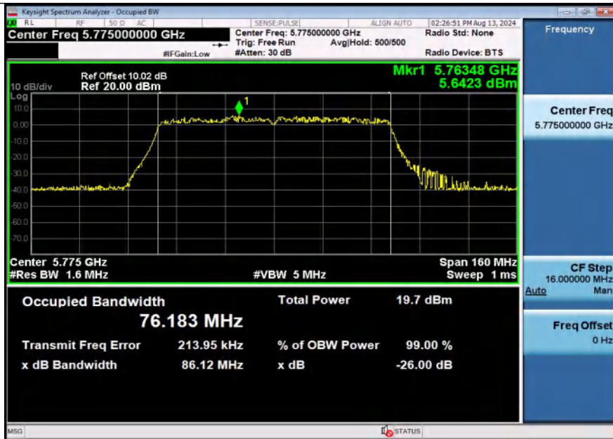
11AC80SISO-Ant2-5775
