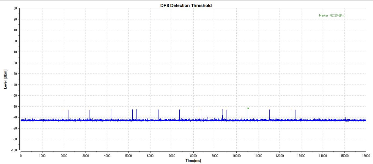
11AX40-5270-Type5-PASS
