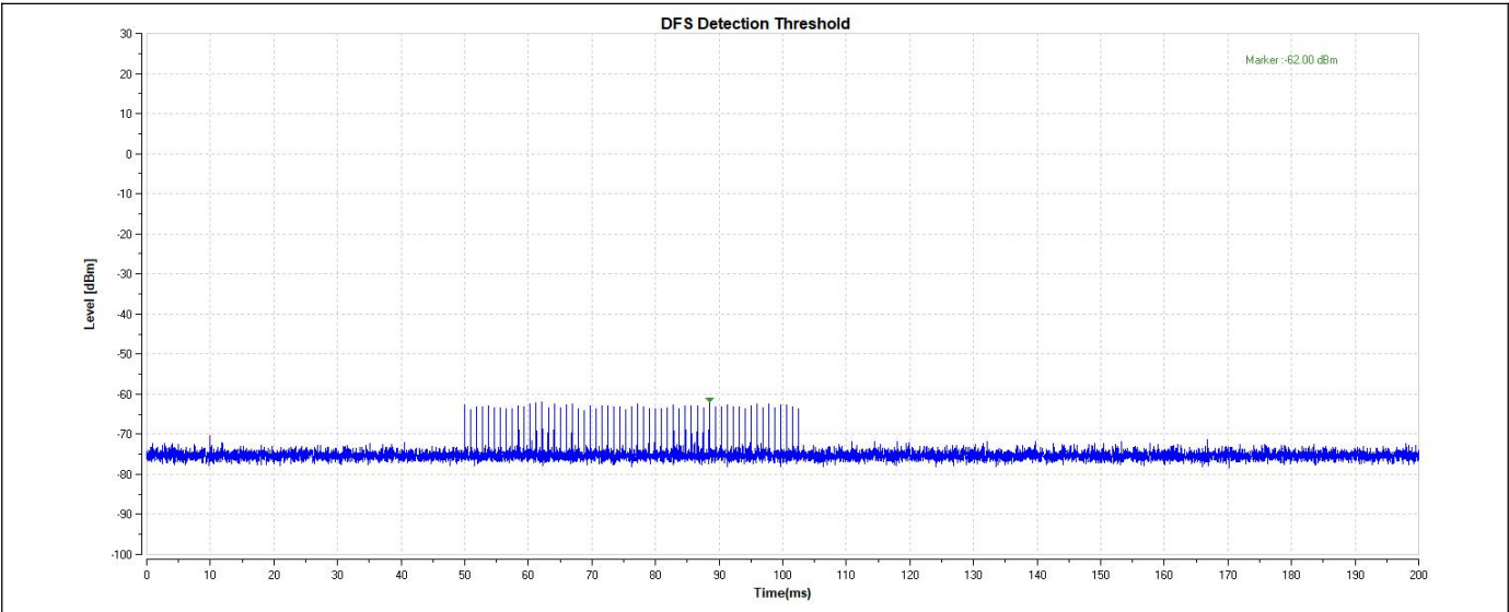
11AX40-5270-Type1-PASS
