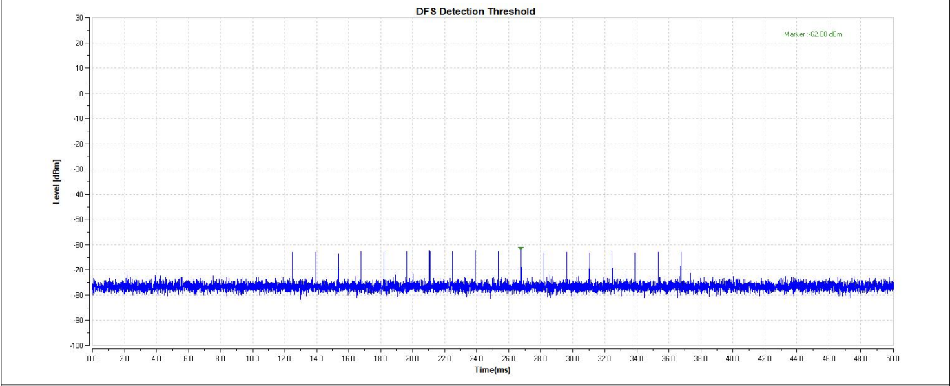
11AX40-5270-Type0-PASS
