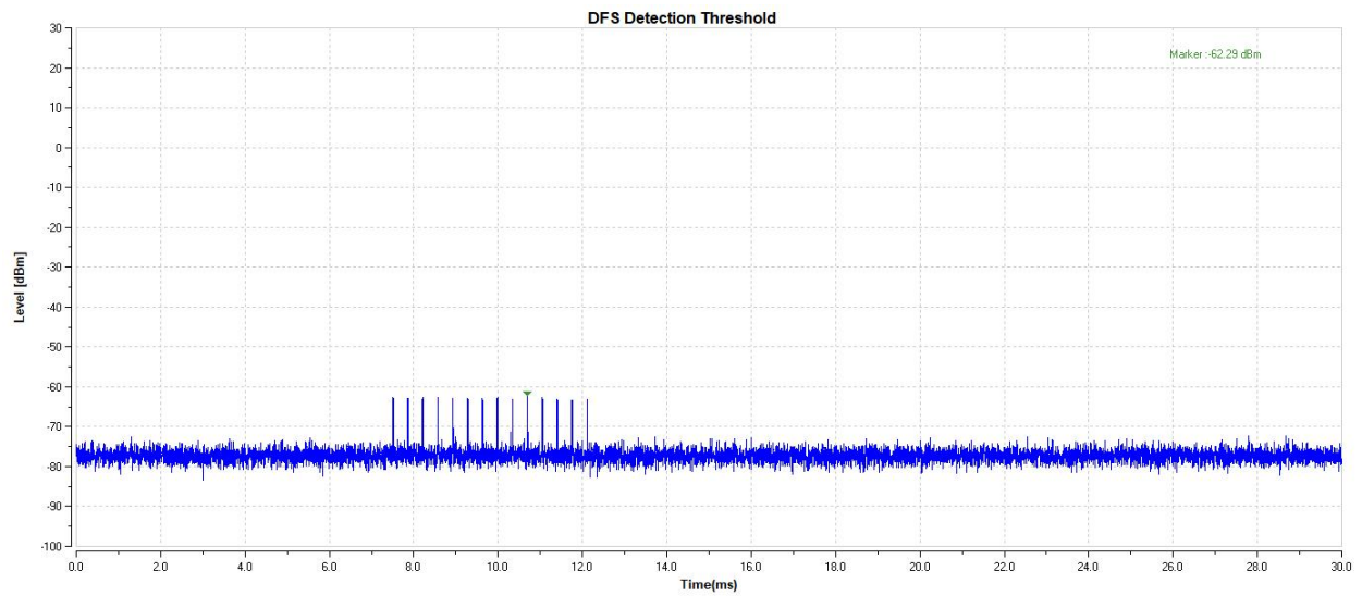
11AX40-5270-Type4-PASS
