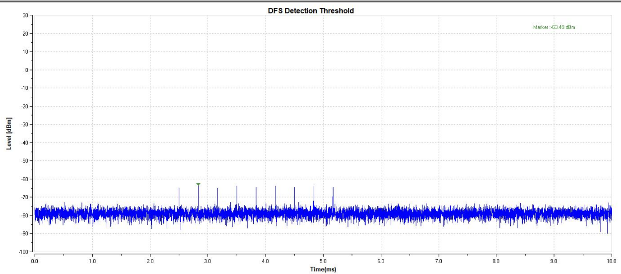
11AX40-5270-Type6-PASS
