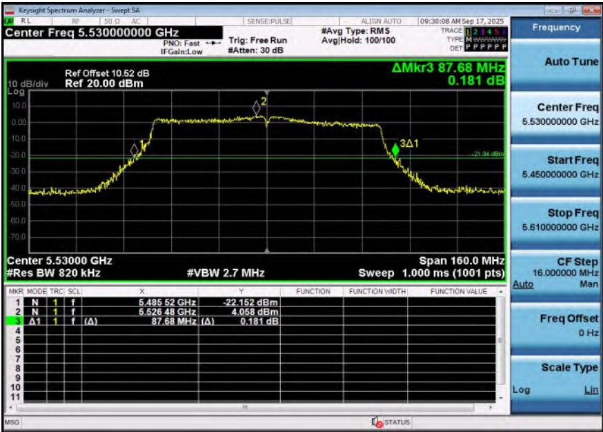
11AC80SISO-Ant1-5530
