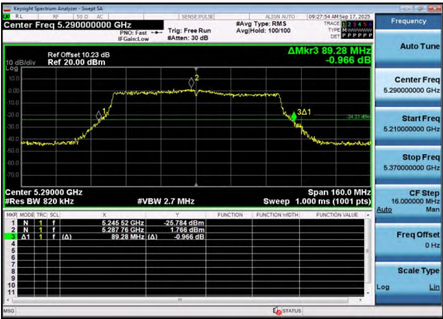
11AC80SISO-Ant1-5290
