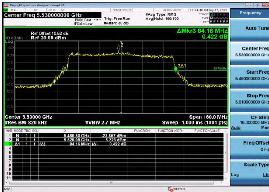
11AX80SISO-Ant1-5530
