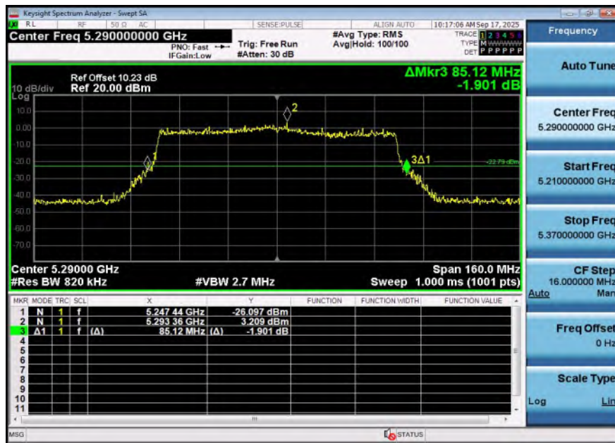
11AX80SISO-Ant1-5290
