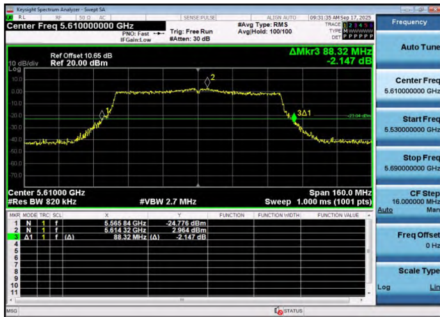
11AC80SISO-Ant1-5610
