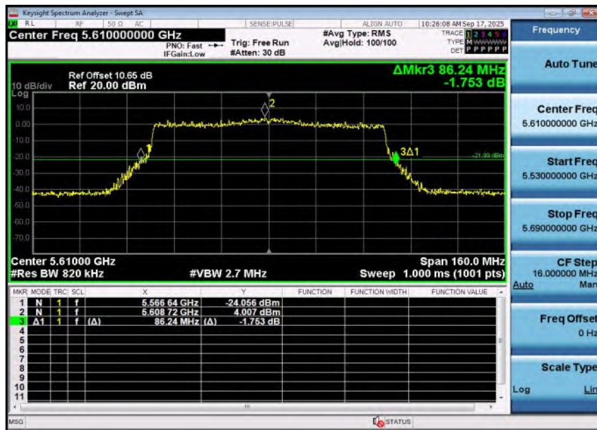
11AX80SISO-Ant1-5610
