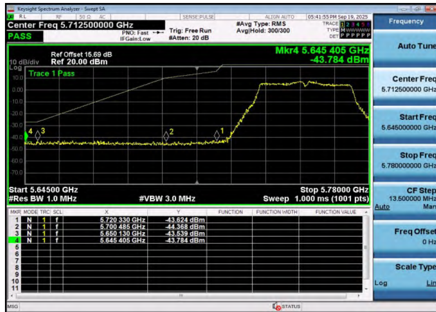
11N40SISO-Ant1-5755-PASS
