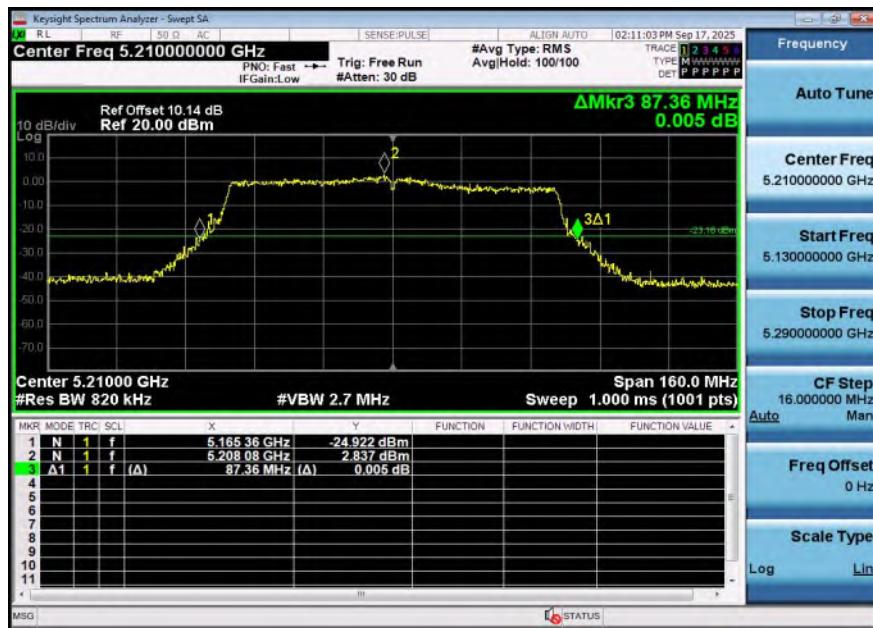
11AC80SISO-Ant2-5210
