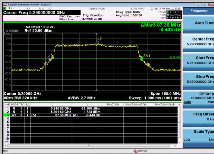
11BE80SISO-Ant1-5290
