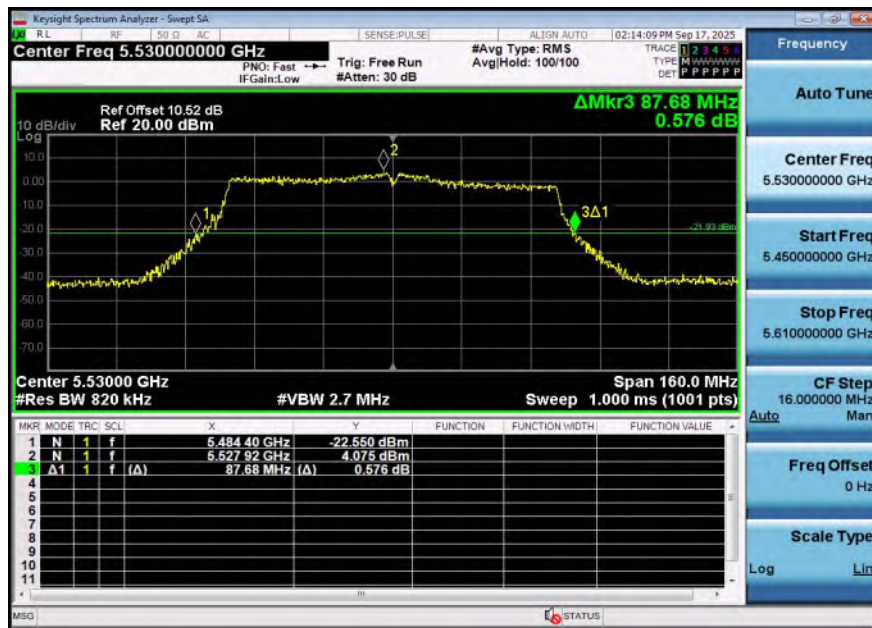
11AC80SISO-Ant2-5530
