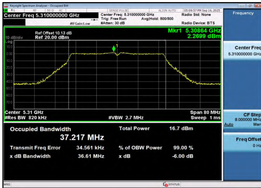
11N40SISO-Ant1-5310
