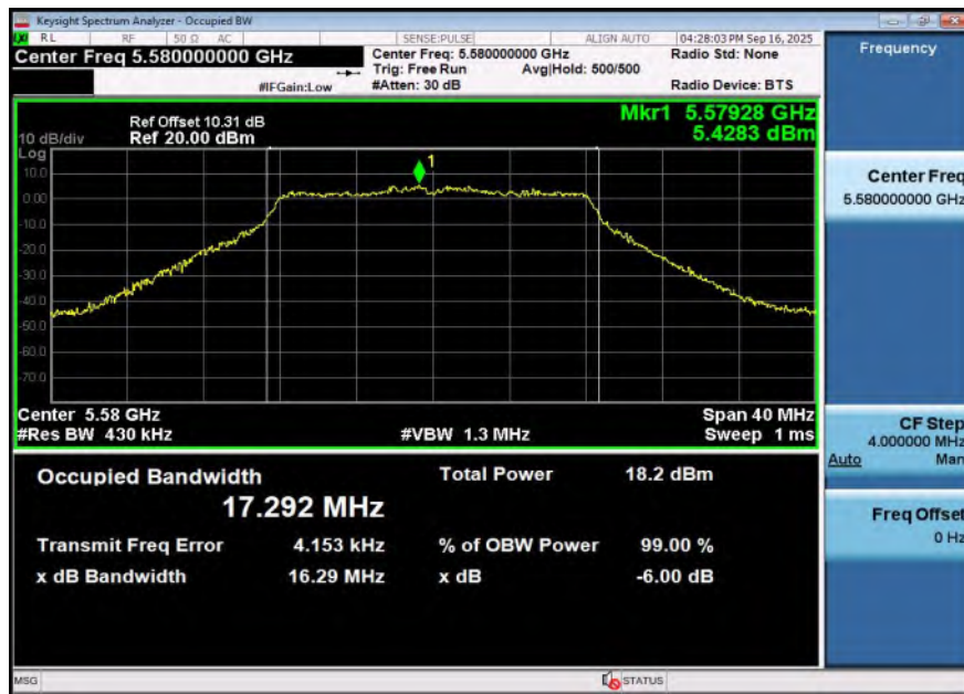
11A-Ant1-5580
