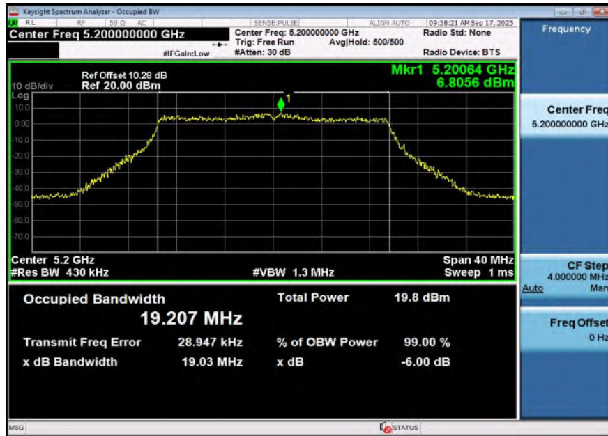
11AX20SISO-Ant1-5200
