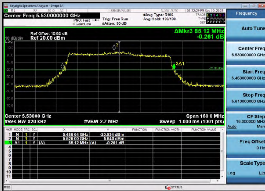
11BE80SISO-Ant2-5530
