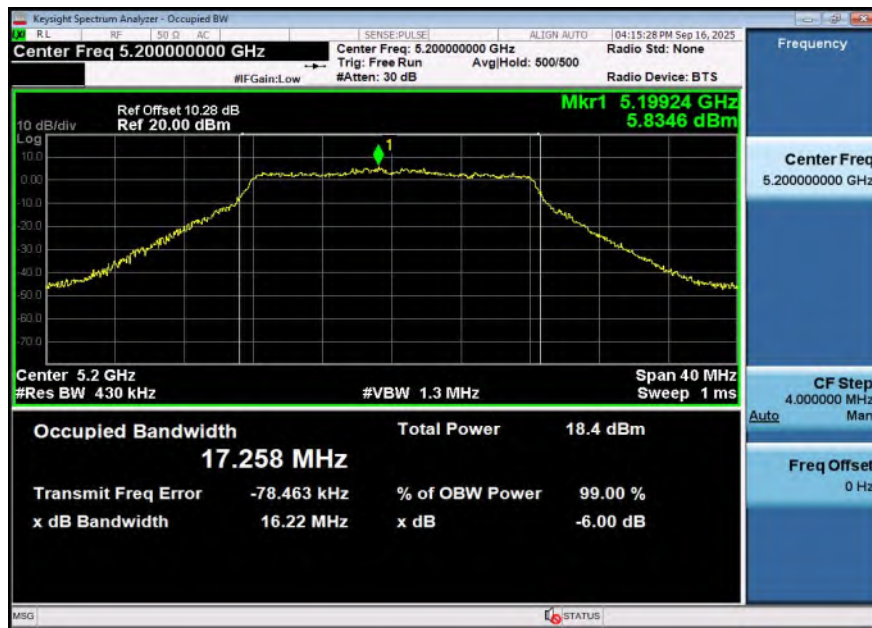
11A-Ant1-5200
