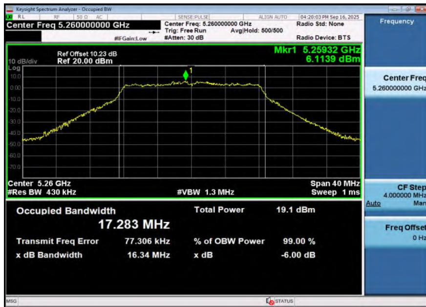
11A-Ant1-5260
