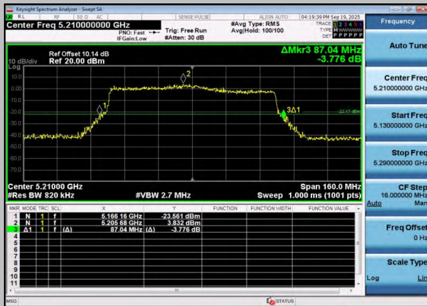
11BE80SISO-Ant2-5210
