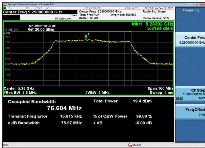
11AC80SISO-Ant1-5290
