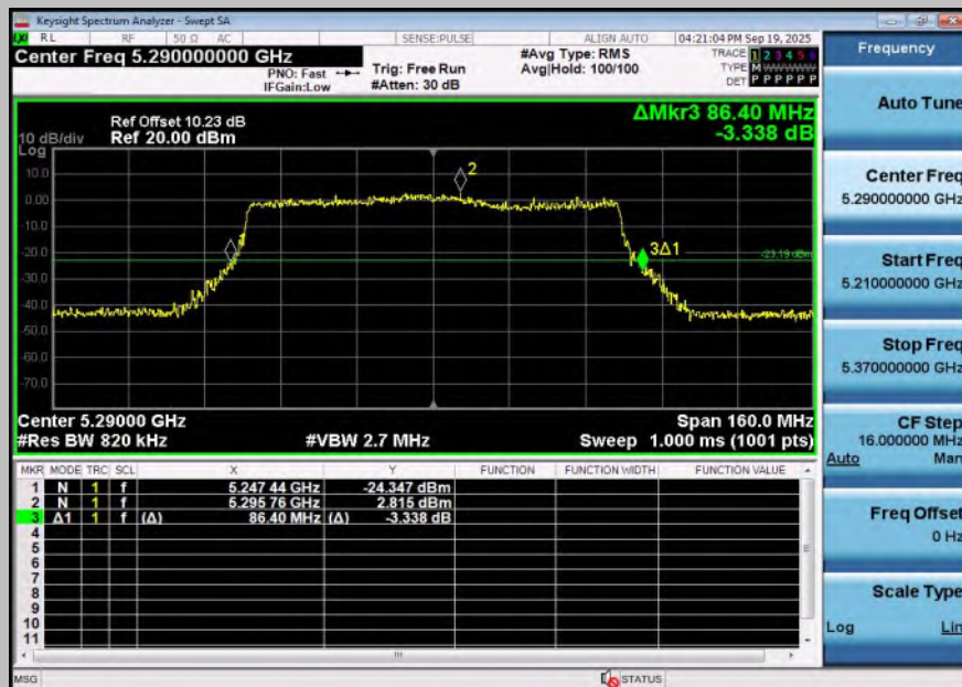
11BE80SISO-Ant2-5290
