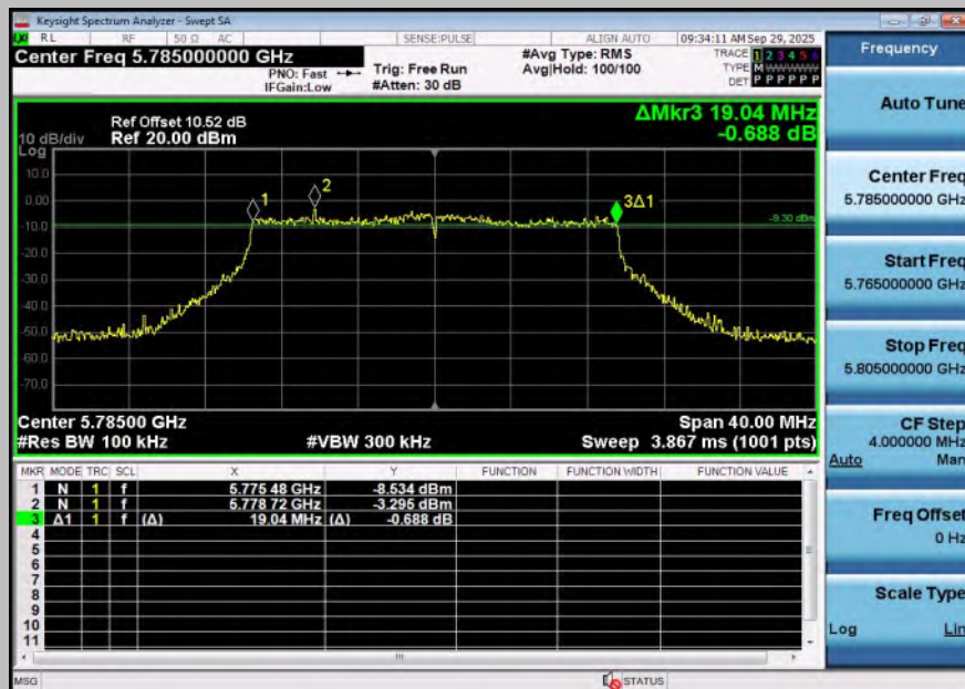
11BE20SISO-Ant1-5785-PASS
