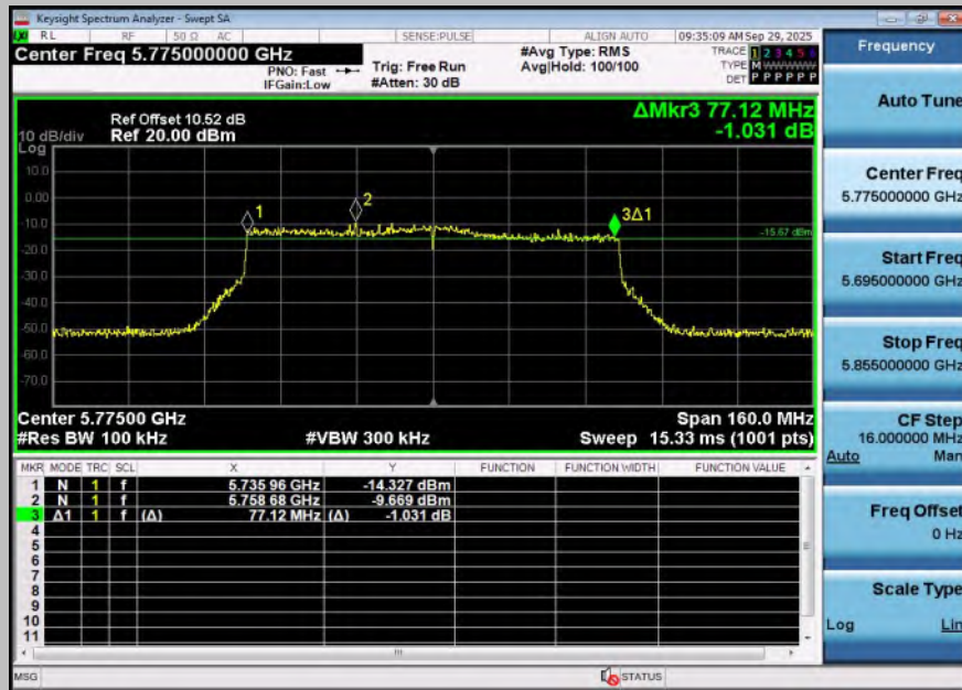
11BE80SISO-Ant1-5775-PASS
