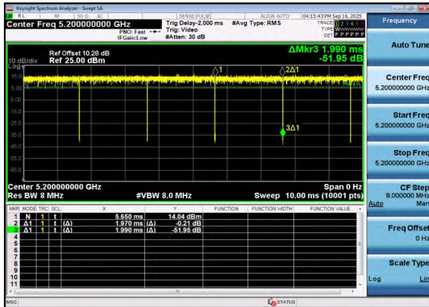
NTNV-11A-Ant1-5200
