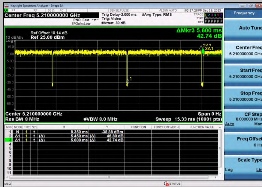
NTNV-11BE80SISO-Ant1-5210
