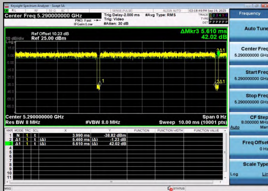
NTNV-11BE80SISO-Ant1-5290
