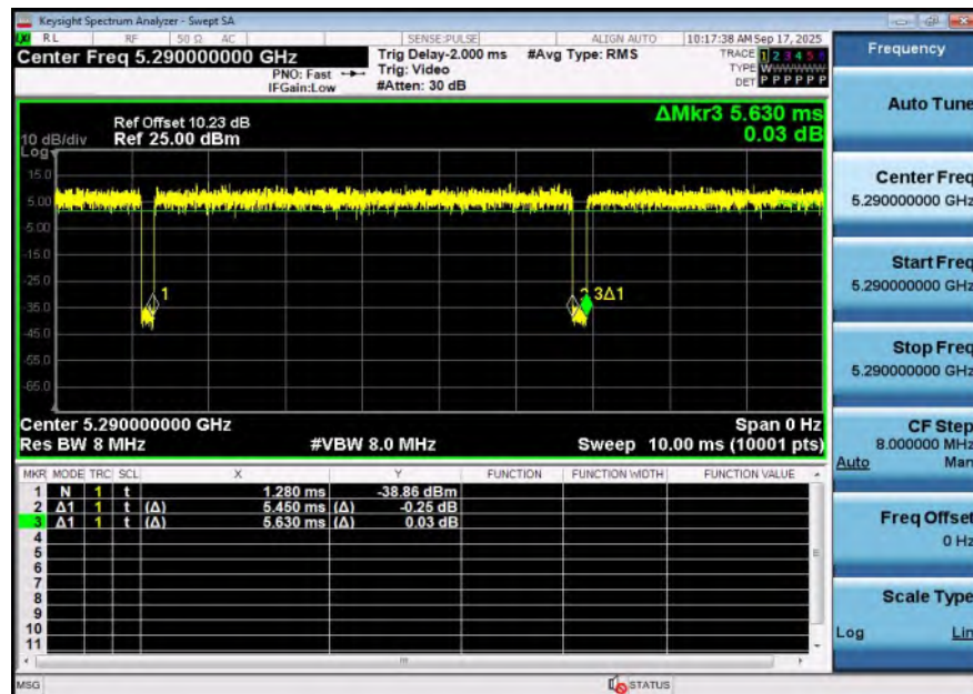
NTNV-11AX80SISO-Ant1-5290
