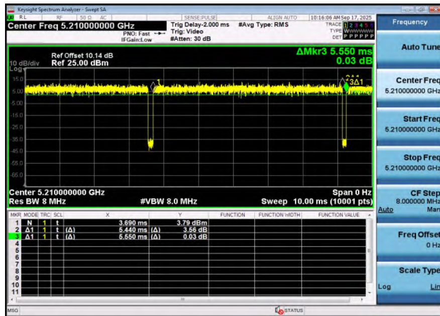
NTNV-11AX80SISO-Ant1-5210
