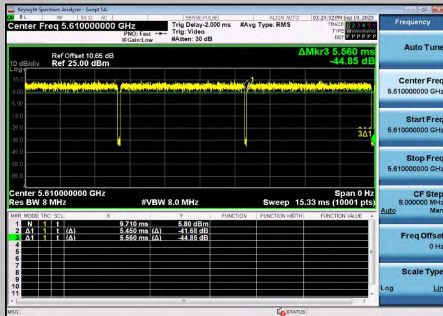
NTNV-11BE80SISO-Ant1-5610
