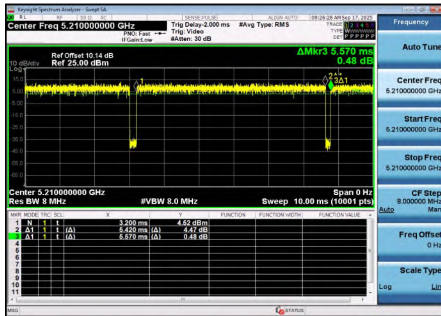
NTNV-11AC80SISO-Ant1-5210
