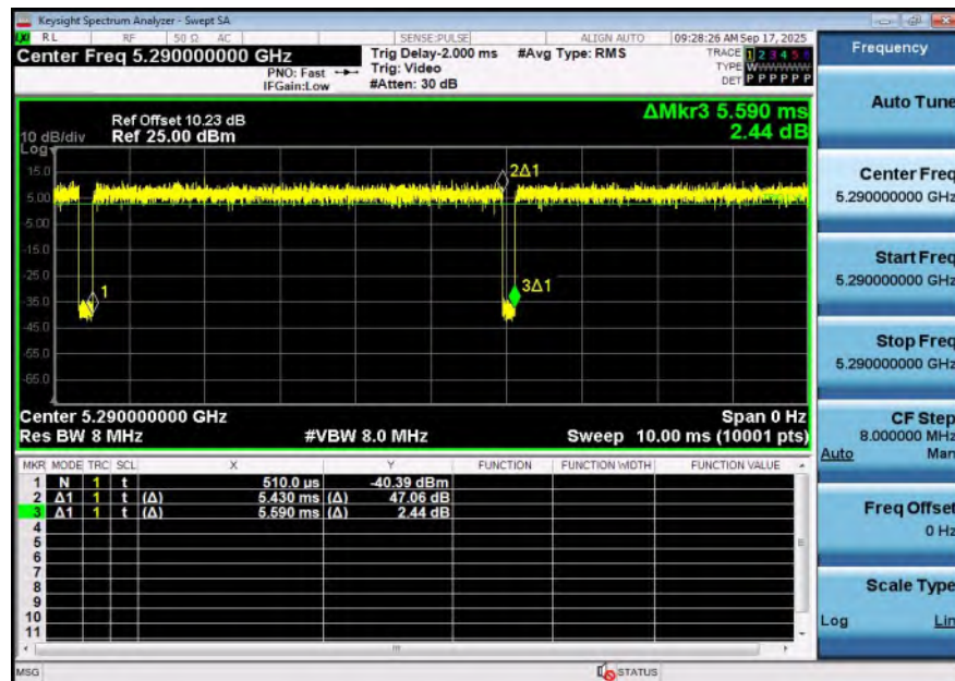
NTNV-11AC80SISO-Ant1-5290
