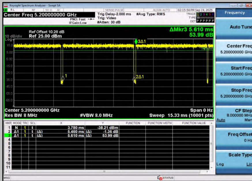
NTNV-11BE20SISO-Ant1-5200
