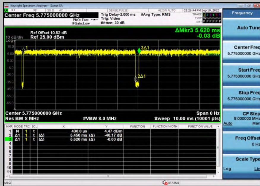
NTNV-11BE80SISO-Ant1-5775
