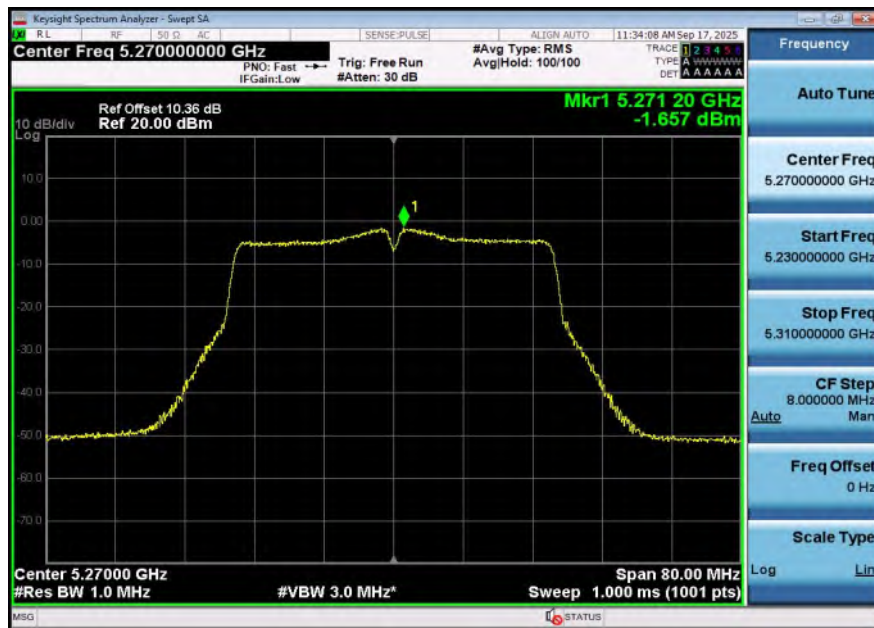
11N40SISO-Ant2-5270-PASS
