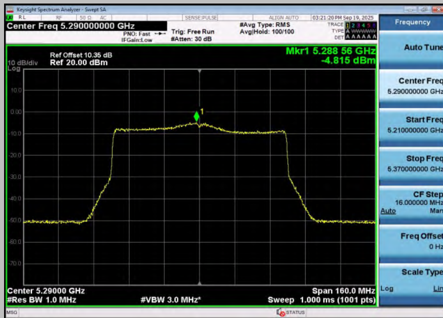
11BE80SISO-Ant1-5290-PASS
