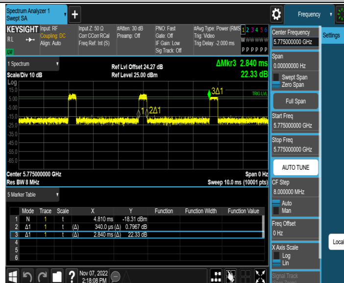
11AX80MIMO_Ant2_5775
