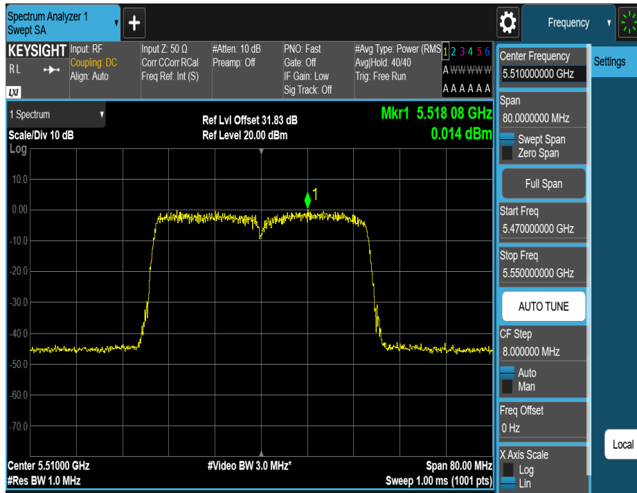
11N40MIMO_Ant2_5510
