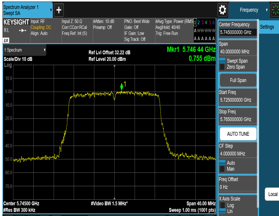
11N20MIMO_Ant2_5745
