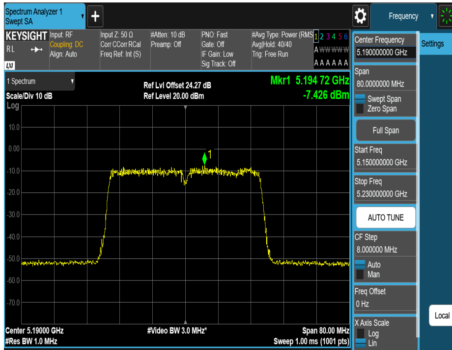
11N40MIMO_Ant2_5190
