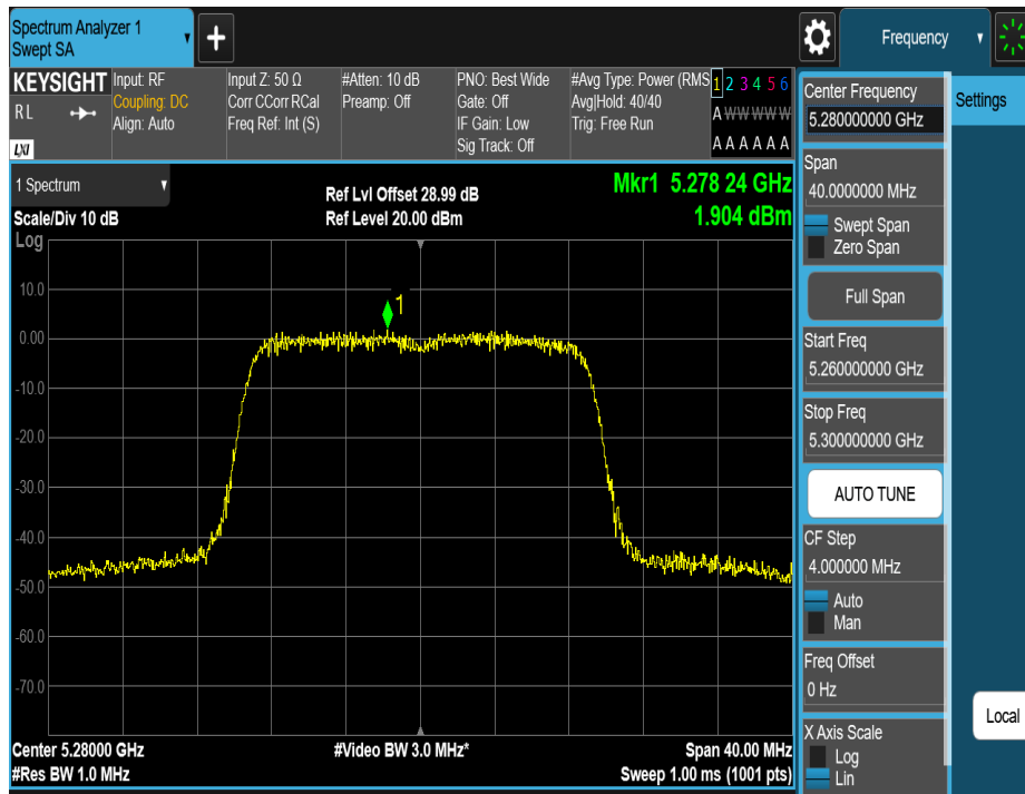
11N20MIMO_Ant2_5280
