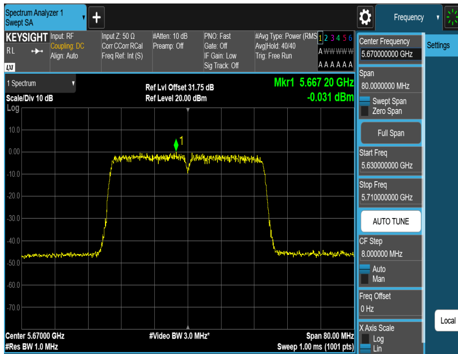
11N40MIMO_Ant2_5670
