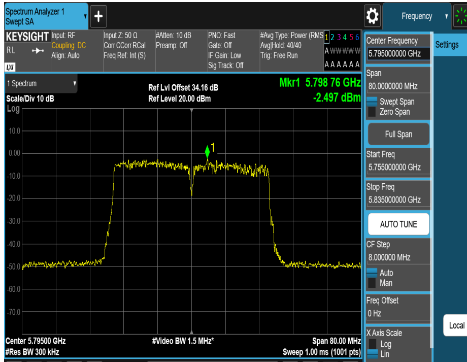
11AC40MIMO_Ant2_5795
