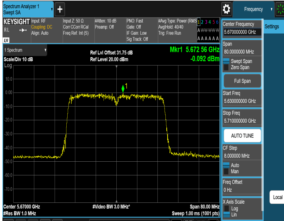
11N40MIMO_Ant2_5670
