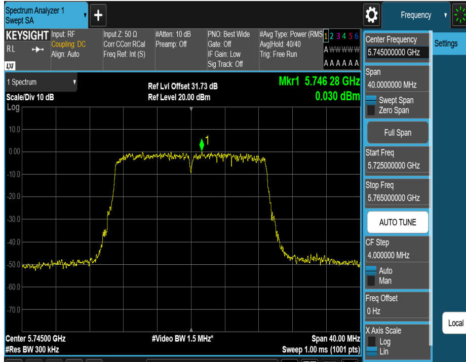
11N20MIMO_Ant2_5745
