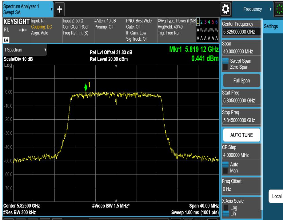
11N20MIMO_Ant2_5825
