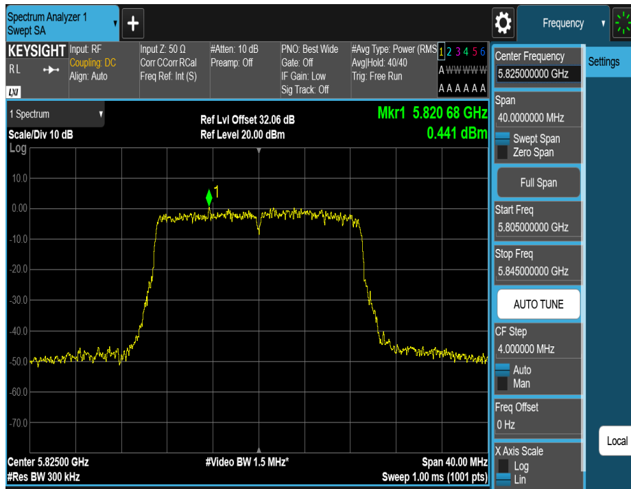
11N20MIMO_Ant2_5825
