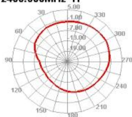
2400.000MHz H
