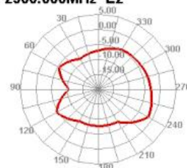
2500.000MHz E2
