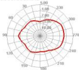
5000.000MHz H
