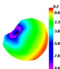
2450.000MHz
