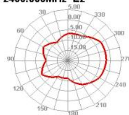
2400.000MHz E2
