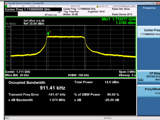
LTE CATM1 B4-5M-Mid CH-OBW-Q16
