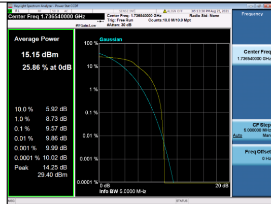
LTE CATM1 B4-20M-High CH-PAPR-Q16
