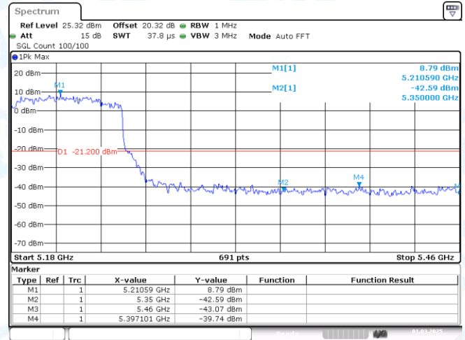
11AX80MIMO-Ant1-5210-PASS
