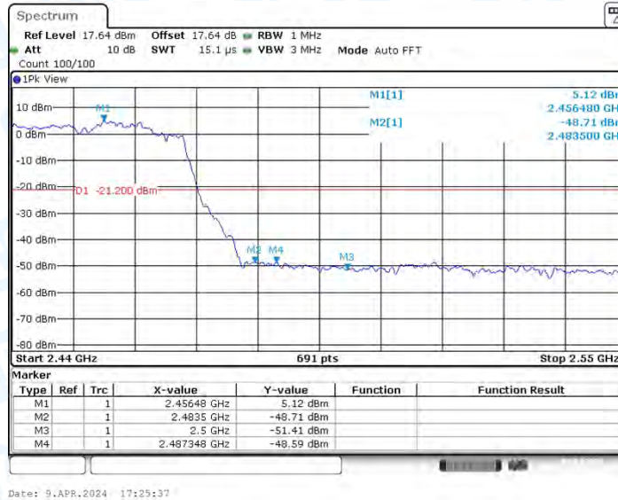
11AX40MIMO_Ant2_High_2452_AV
