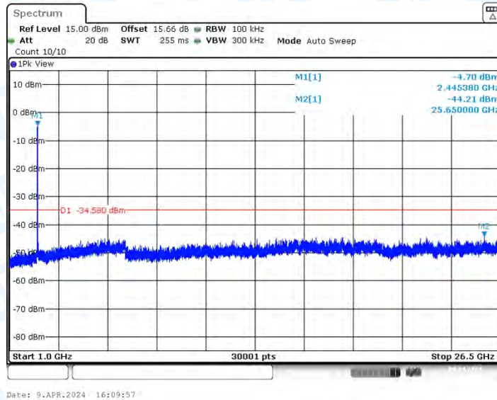
11N40MIMO_Ant2_2437_0~Reference
