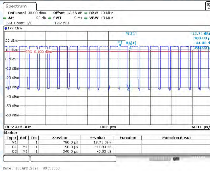
11G-CDD_Ant2_2412
