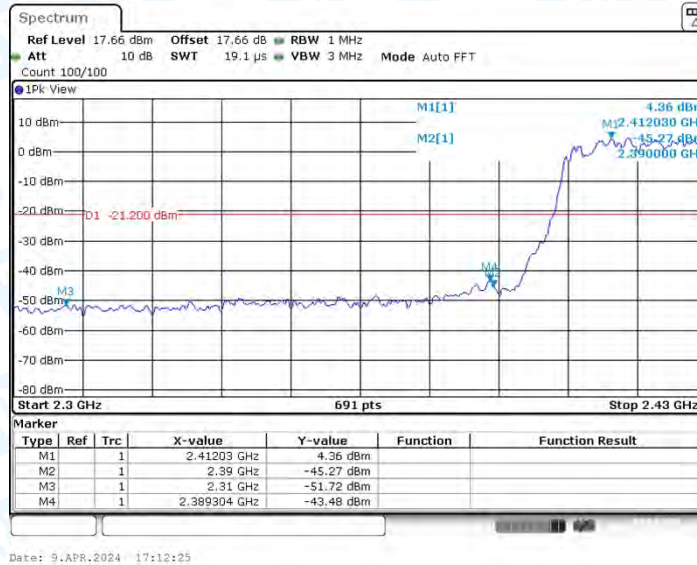
11AX40MIMO_Ant2_Low_2422_AV
