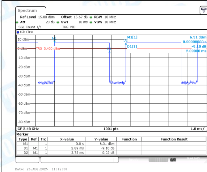
NTNV-DH5-Ant1-2480
