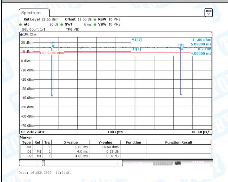
NTVN-11AX20MIMO-Ant1-2437
