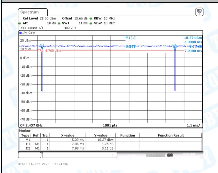
NTNV-11N40MIMO-Ant1-2437
