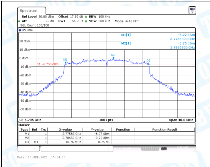
11AX20MIMO-Ant1-5785-PASS
