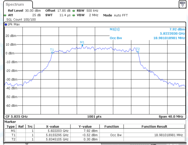
11AX20MIMO-Ant2-5825
