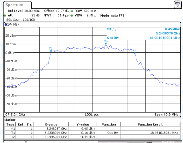
11AX20MIMO-Ant2-5240
