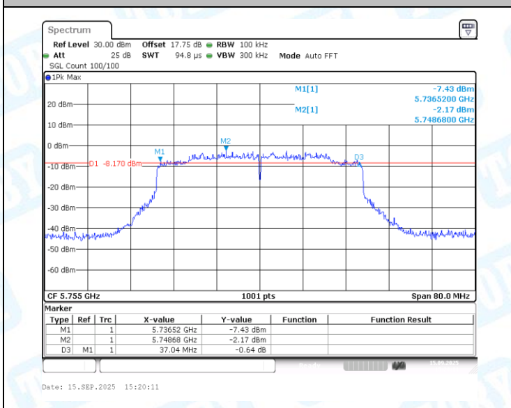
11AX40MIMO-Ant1-5755-PASS
