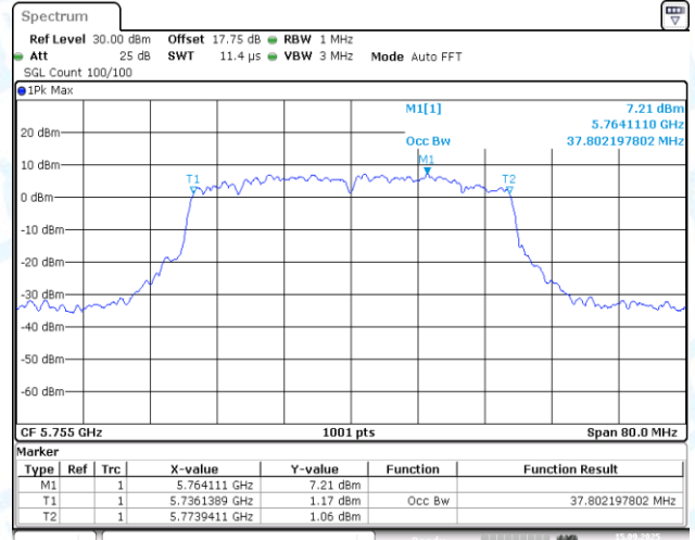
11AX40MIMO-Ant2-5755
