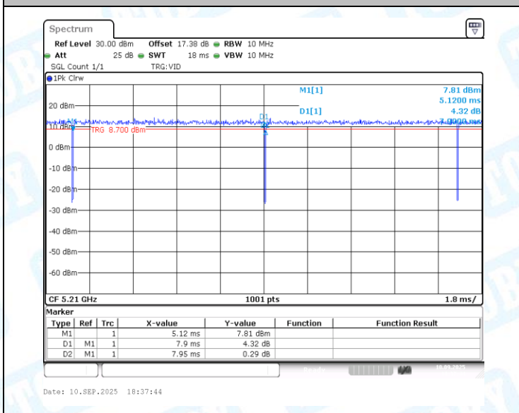
NTNV-11AC80MIMO-Ant1-5210
