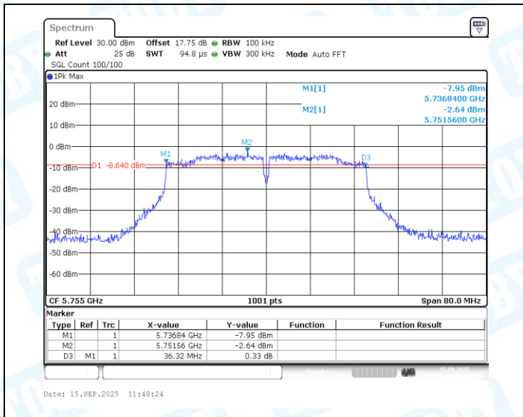
11N40MIMO-Ant1-5755-PASS
