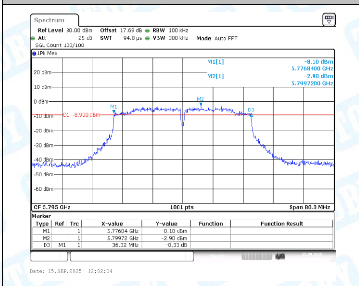
11N40MIMO-Ant1-5795-PASS
