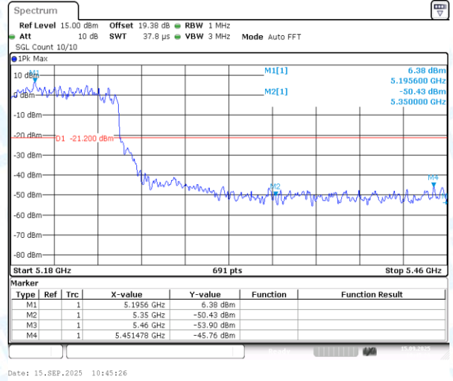
11AX80MIMO-Ant1-5210-PASS
