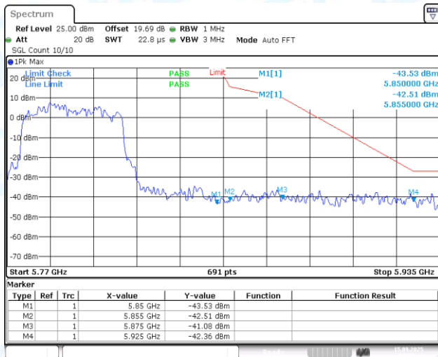
11AX40MIMO-Ant1-5755-PASS
