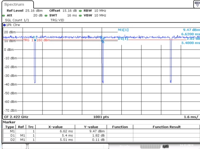
NTNV-11AX40MIMO-Ant1-2422
