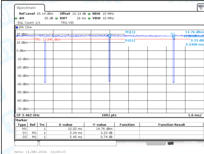
NTNV-11AX20MIMO-Ant1-2462
