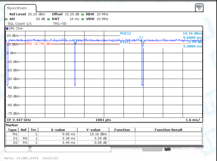
NTNV-11N40MIMO-Ant2-2437
