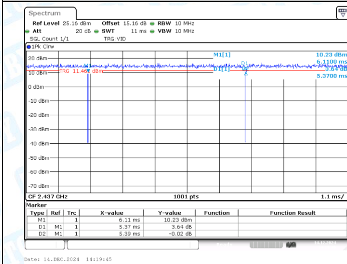
NTNV-11N40MIMO-Ant1-2437
