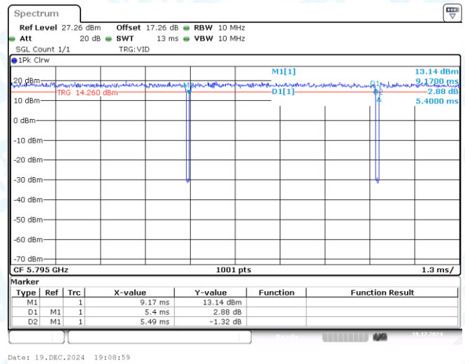
NTNV-11AX40MIMO-Ant2-5795
