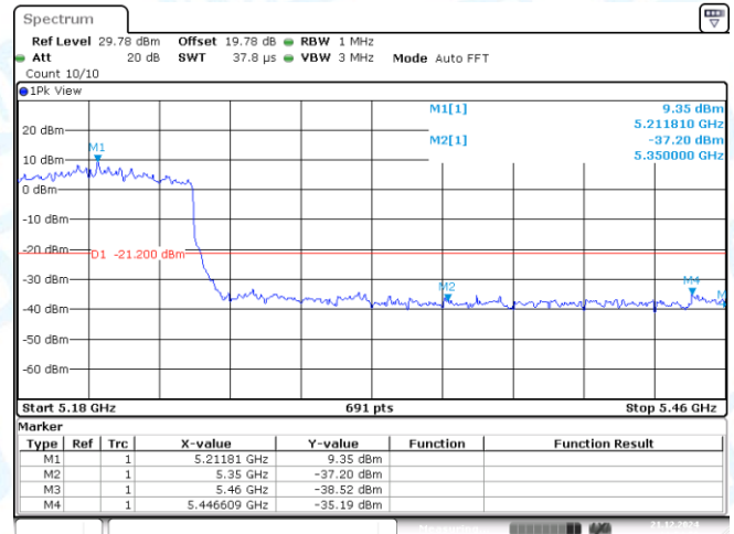
11AX80MIMO-Ant1-5210-PASS
