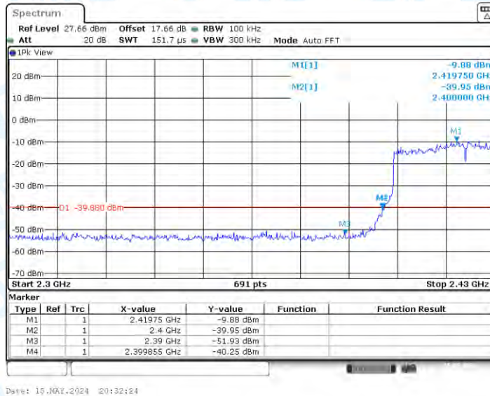
11AX40MIMO_Ant2_Low_2422
