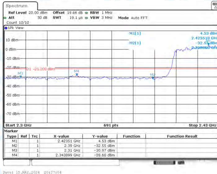
11AX40MIMO_Ant2_Low_2422_AV
