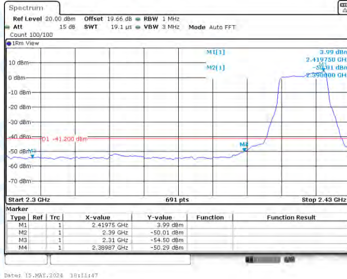
11N20MIMO_Ant1_Low_2412_Peak
