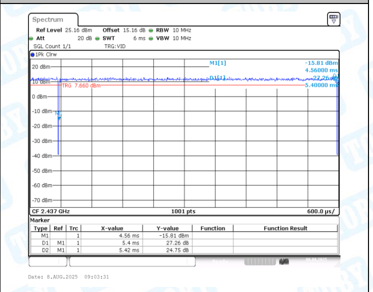
NTNV-11N20MIMO-Ant1-2437
