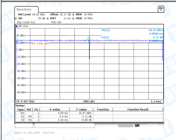
NTNV-11N20MIMO-Ant2-2437
