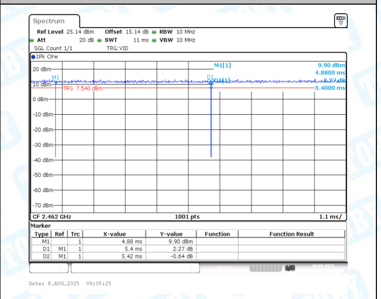
NTNV-11N20MIMO-Ant1-2462
