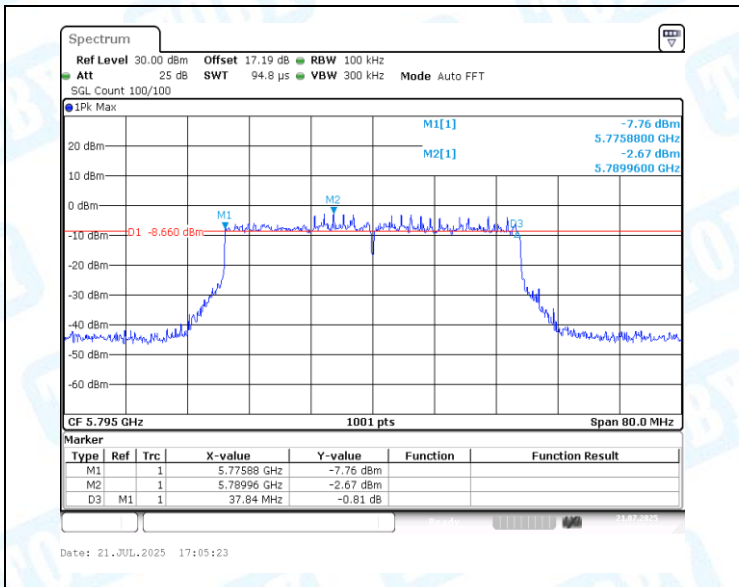
11AX40MIMO-Ant1-5795-PASS
