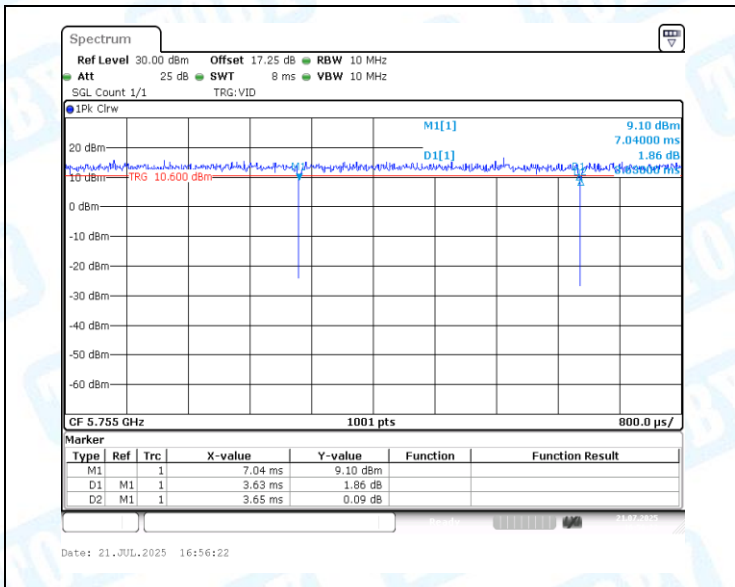
NTNV-11AX40MIMO-Ant1-5755
