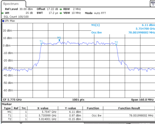
11AX80MIMO-Ant1-5775
