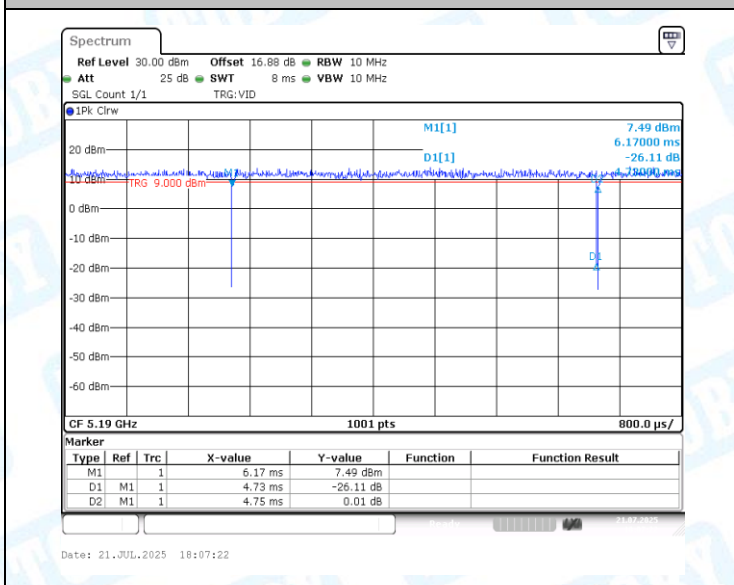
NTNV-11N40MIMO-Ant1-5190
