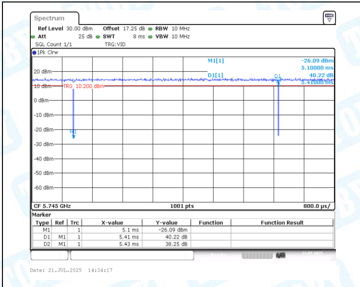
NTNV-11N20MIMO-Ant1-5745
