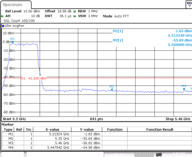
11AX40MIMO-Ant1-5230-PASS
