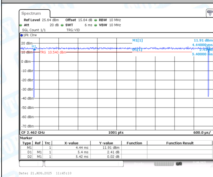
NTNV-11N20MIMO-Ant1-2462
