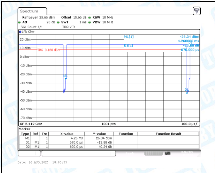
NTVN-11B-CDD-Ant1-2412
