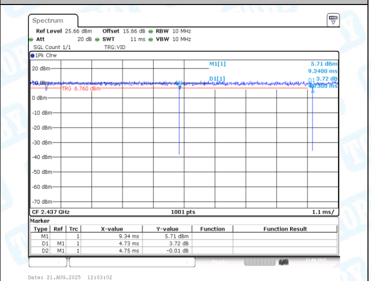
NTNV-11N40MIMO-Ant1-2437
