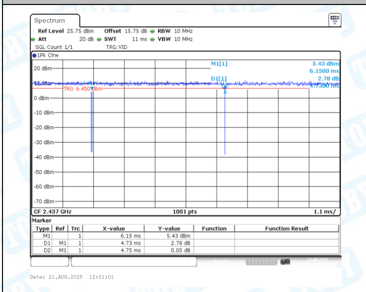
NTNV-11N40MIMO-Ant2-2437
