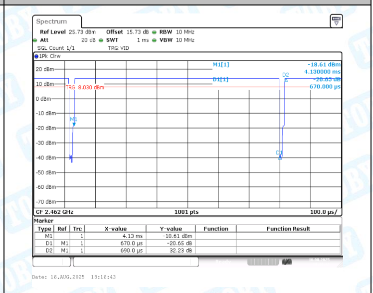
NTVN-11B-CDD-Ant2-2462
