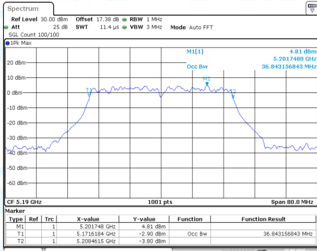
11N40MIMO-Ant1-5190
