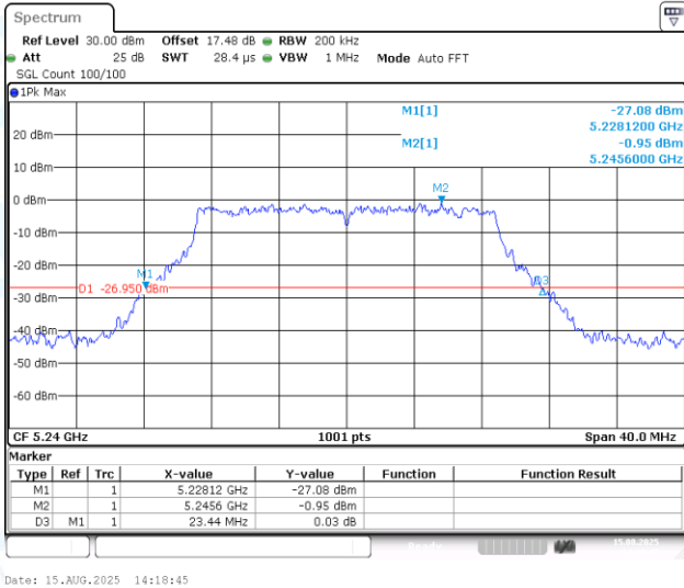
11N20MIMO-Ant1-5240
