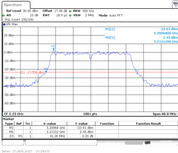
11AC40MIMO-Ant1-5230
