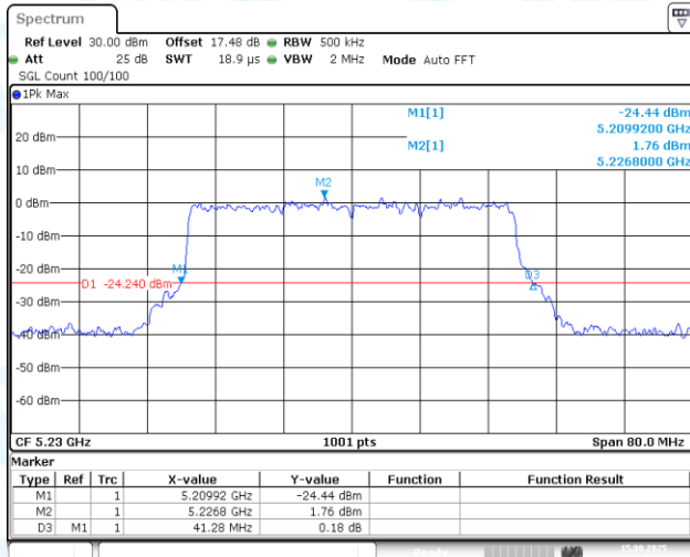
11AX40MIMO-Ant1-5230
