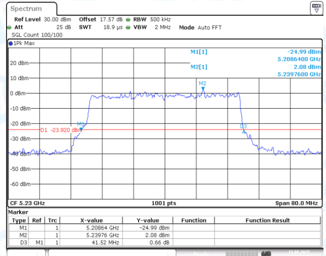
11AX40MIMO-Ant2-5230
