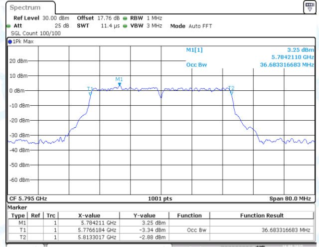
11N40MIMO-Ant2-5795
