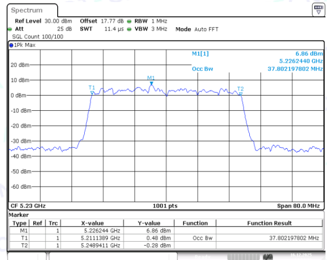
11AX40MIMO-Ant2-5230
