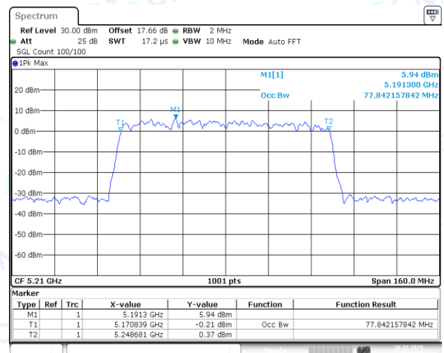
11AX80MIMO-Ant2-5210
