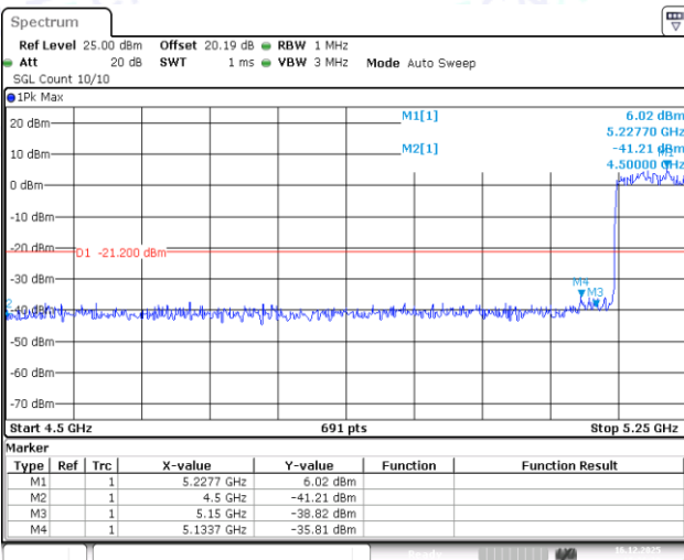
11AX80MIMO-Ant1-5210-PASS
