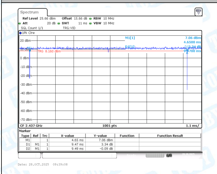
NTNV-11N40MIMO-Ant1-2437
