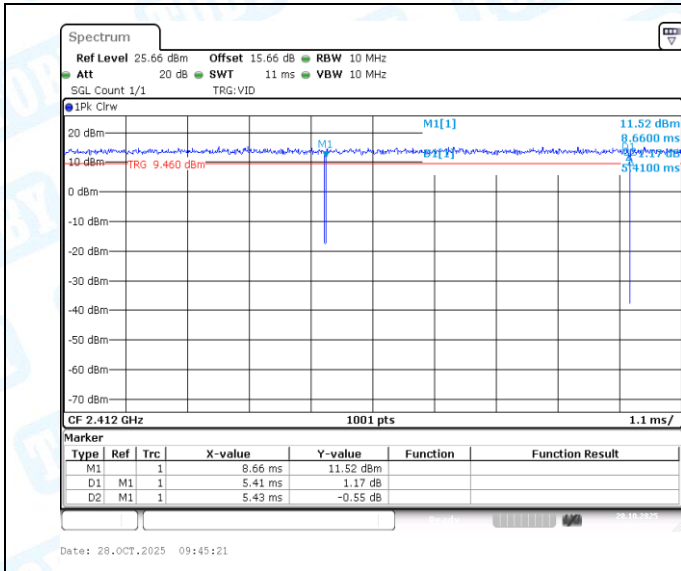
NTNV-11AX20MIMO-Ant1-2412
