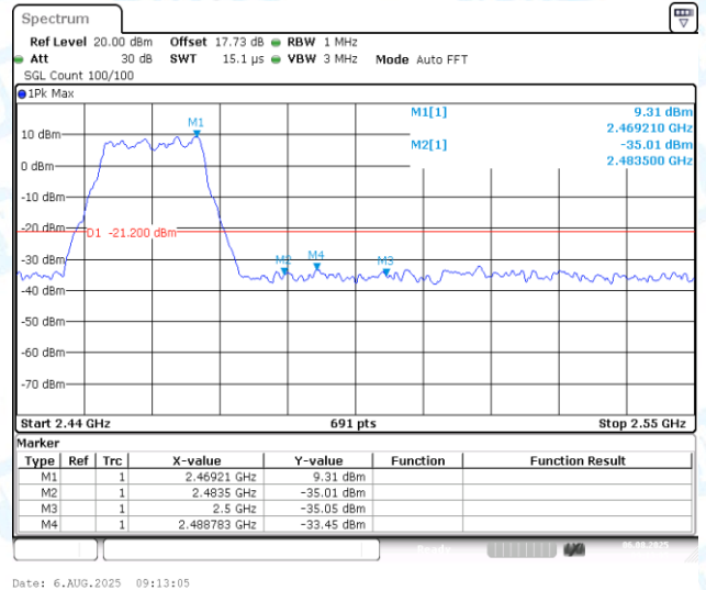
11G-CDD-Ant2-2462-PASS
