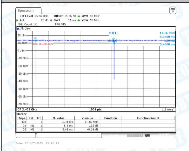
NTNV-11N20MIMO-Ant1-2437
