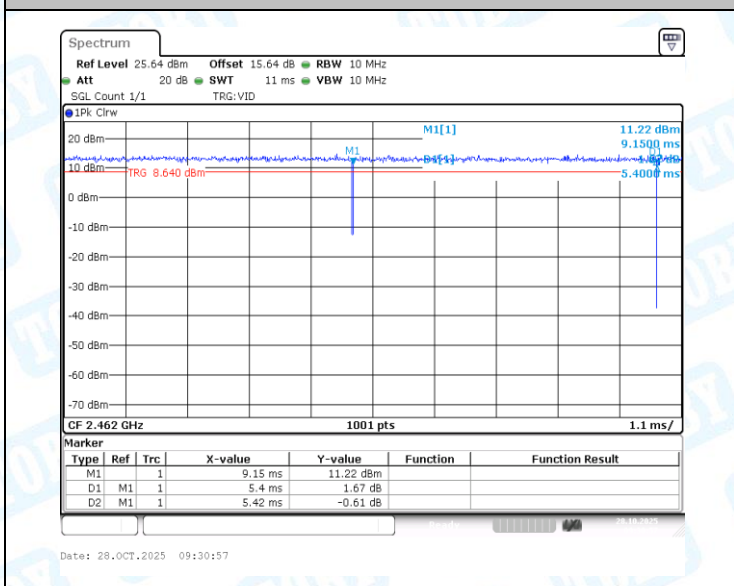
NTNV-11N20MIMO-Ant1-2462
