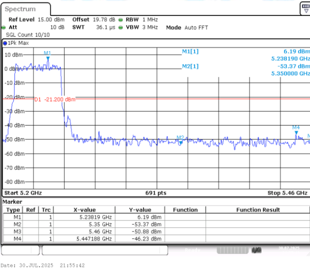
11AX40MIMO-Ant1-5230-PASS
