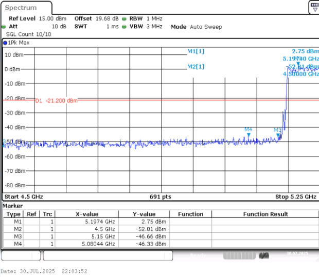
11AX80MIMO-Ant1-5210-PASS
