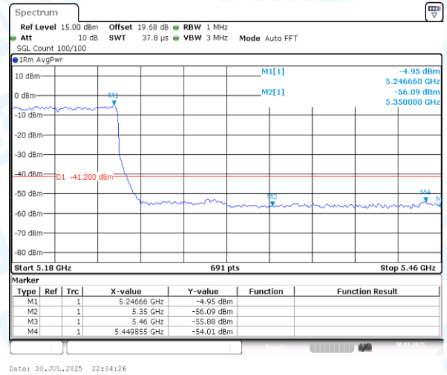
11AX80MIMO-Ant1-5210-PASS
