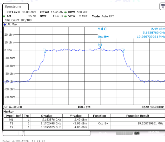
11AX20MIMO-Ant1-5180
