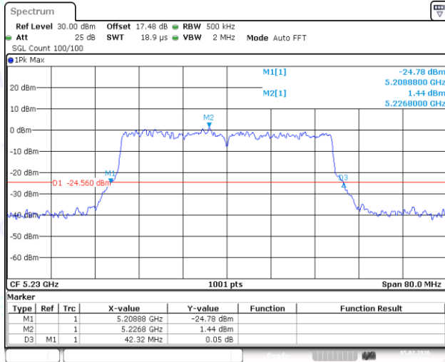
11AX40MIMO-Ant1-5230
