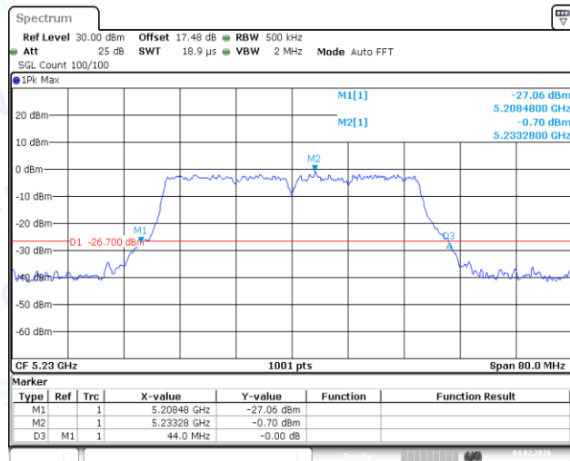
11AC40MIMO-Ant1-5230
