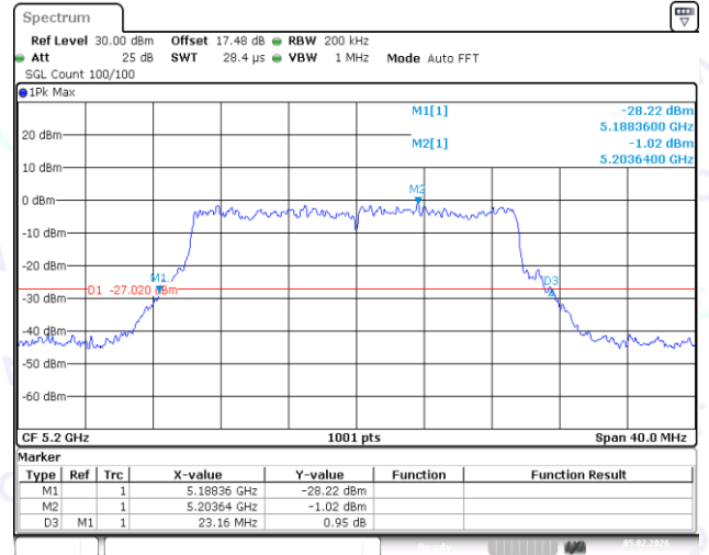
11AX20MIMO-Ant2-5200
