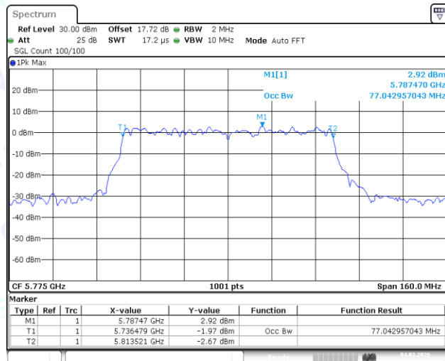
11AC80MIMO-Ant1-5775
