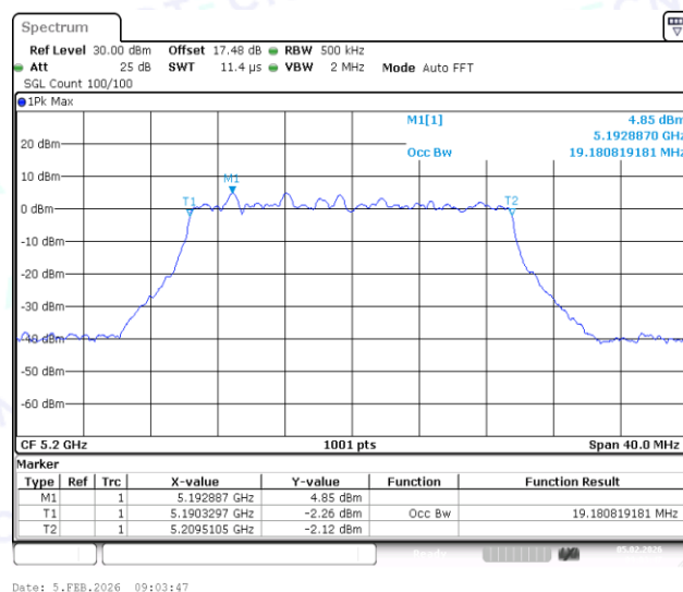
11AX20MIMO-Ant2-5200
