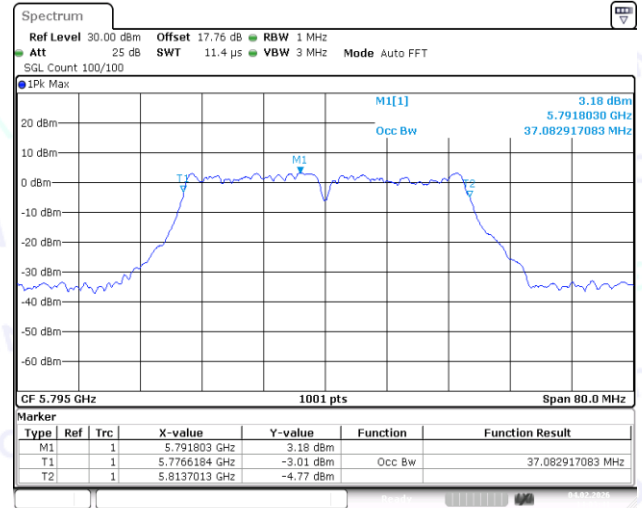
11N40MIMO-Ant2-5795
