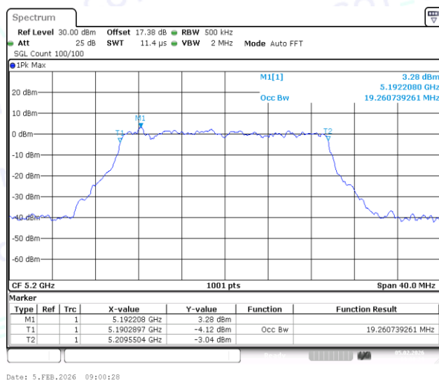
11AX20MIMO-Ant1-5200
