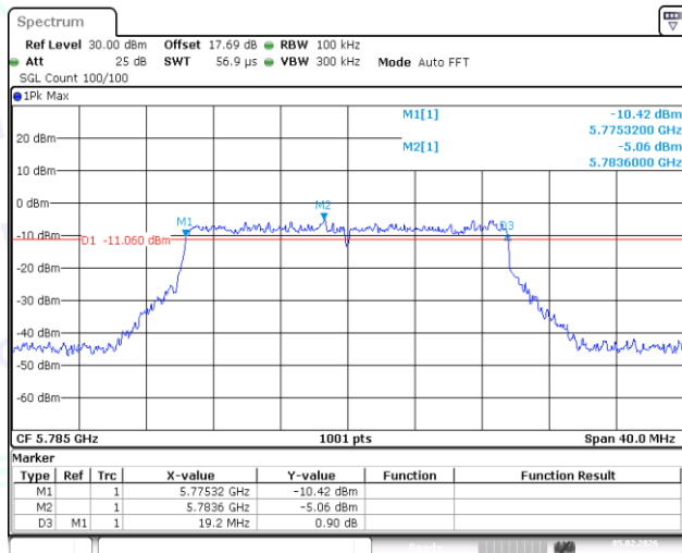
11AX20MIMO-Ant1-5785-PASS
