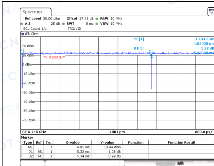
NTNV-11N20MIMO-Ant1-5745
