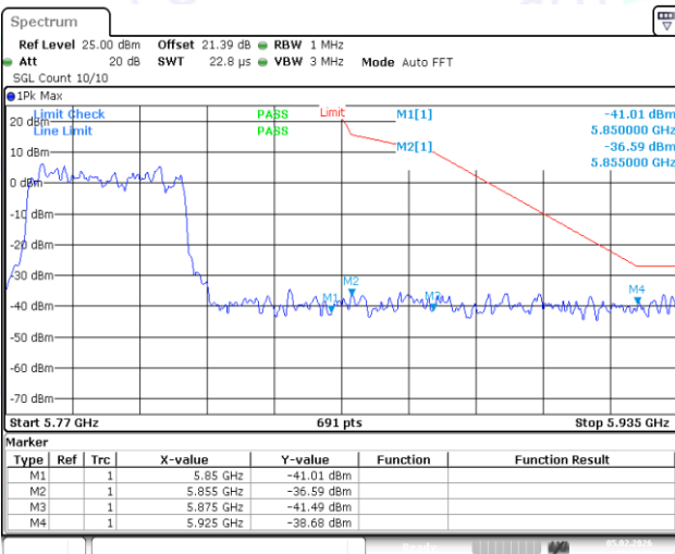
11AX40MIMO-Ant1-5755-PASS
