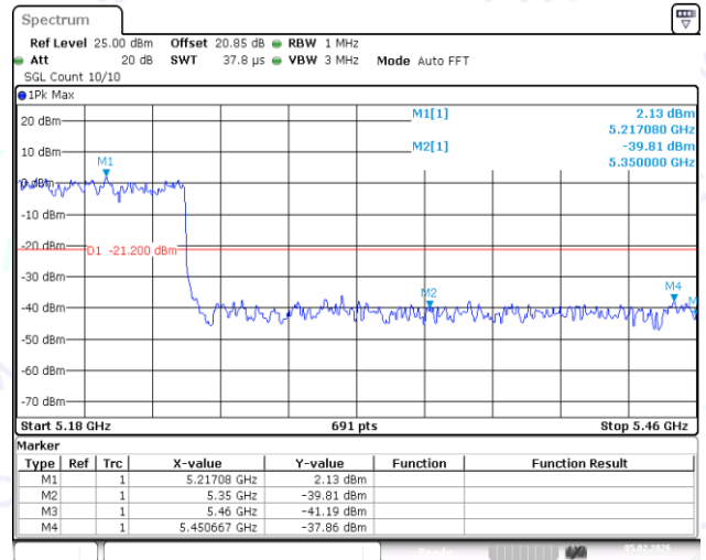
11AX80MIMO-Ant1-5210-PASS
