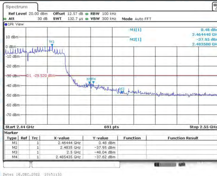
11AX40MIMO_Ant2_High_2452
