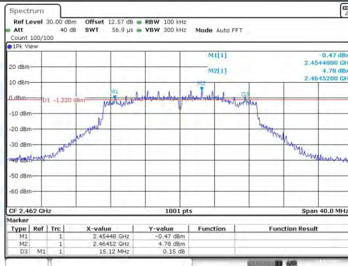
11N20MIMO_Ant2_2462
