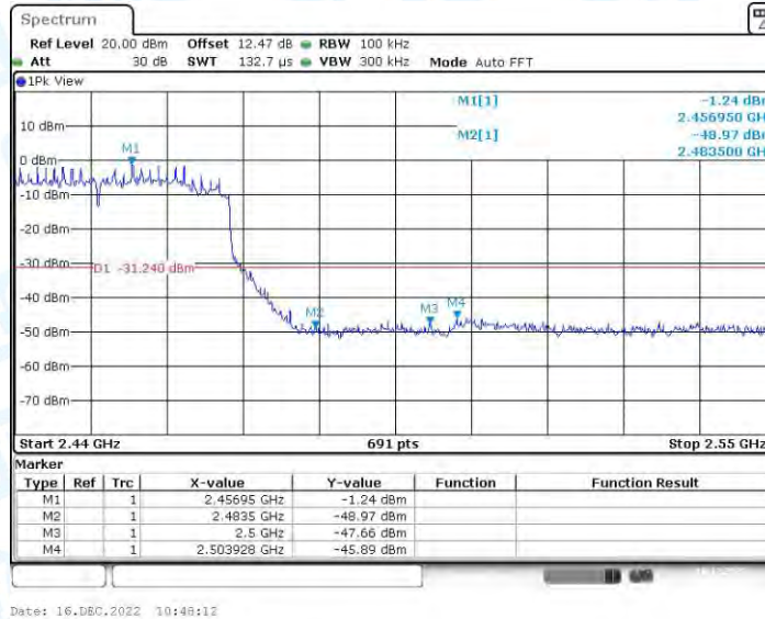
11AX40MIMO_Ant2_High_2452
