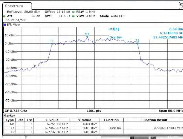
11AX40MIMO_Ant1_5755
