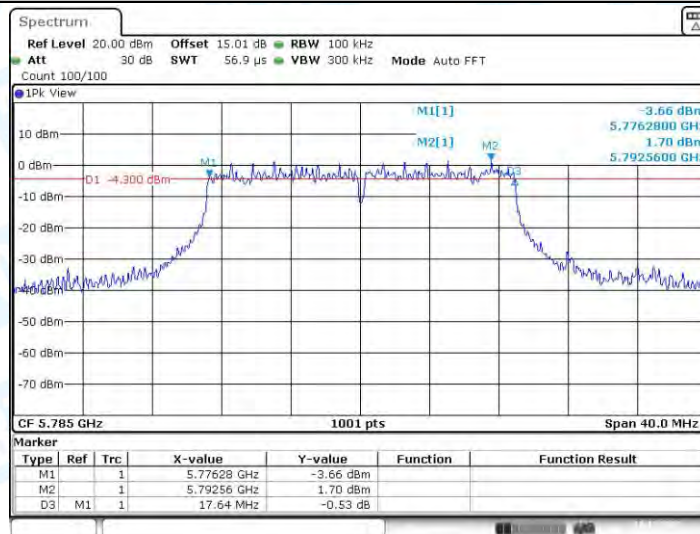
11AC20MIMO_Ant2_5785
