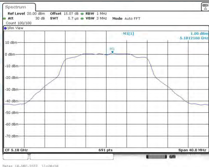
11A-CDD_Ant2_5180
