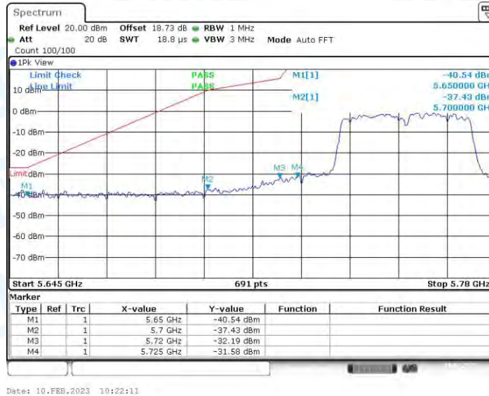
11AX40MIMO_Ant2_Low_5755_Peak
