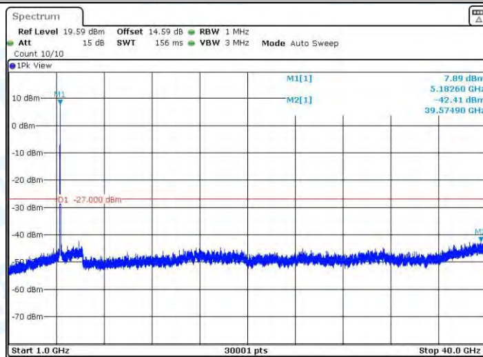
11AC40MIMO_Ant2_5190_1000~40000
