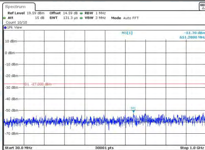
11AC40MIMO_Ant2_5190_30~1000
