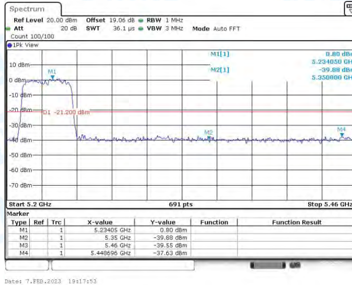
11AX40MIMO_Ant2_High_5230_AV
