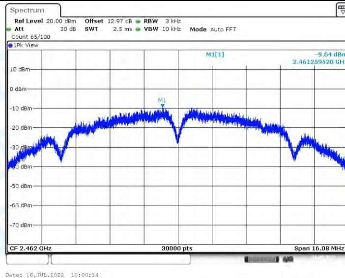
11B-CDD_Ant0_2462
