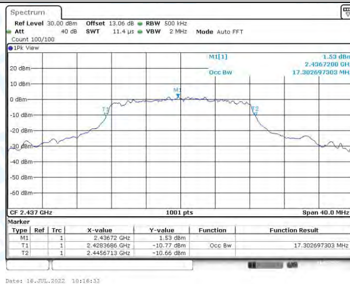
11G-CDD_Ant0_2437
