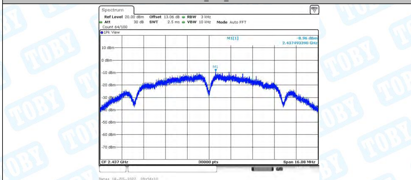
11B-CDD_Ant0_2437
