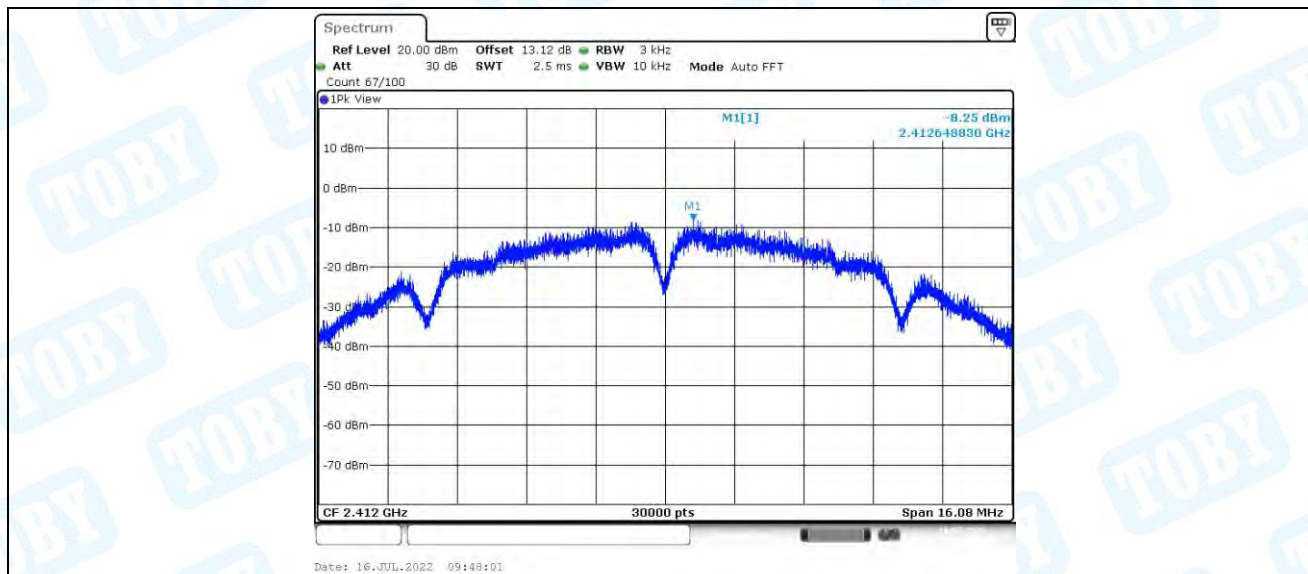
11B-CDD_Ant0_2412
