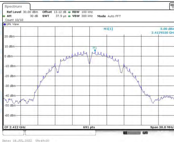
11B-CDD_Ant0_2412_0~Reference
