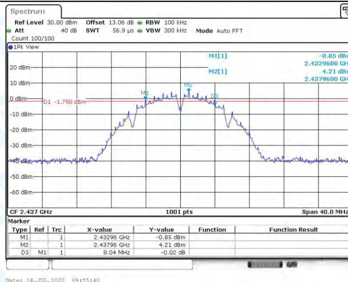
11B-CDD_Ant0_2437
