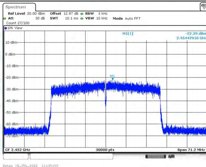
11AX40MIMO_Ant0_2452
