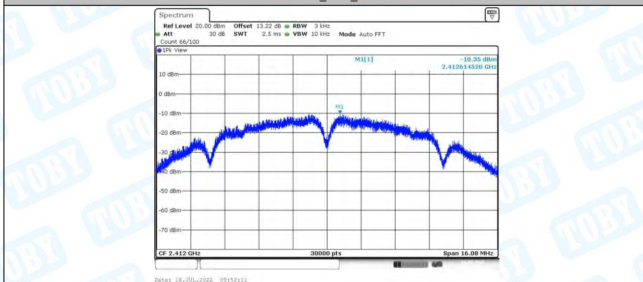
11B-CDD_Ant1_2412
