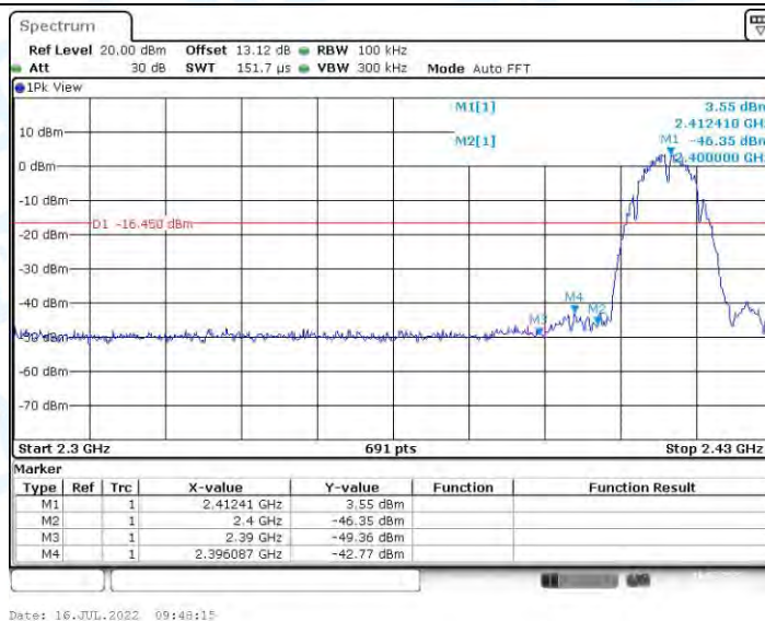
11B-CDD_Ant0_Low_2412
