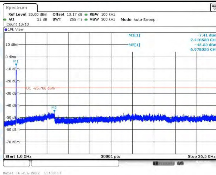
11AX40MIMO_Ant1_2422_1000~26500
