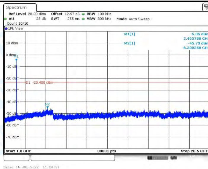
11AX20MIMO_Ant0_2462_1000~26500
