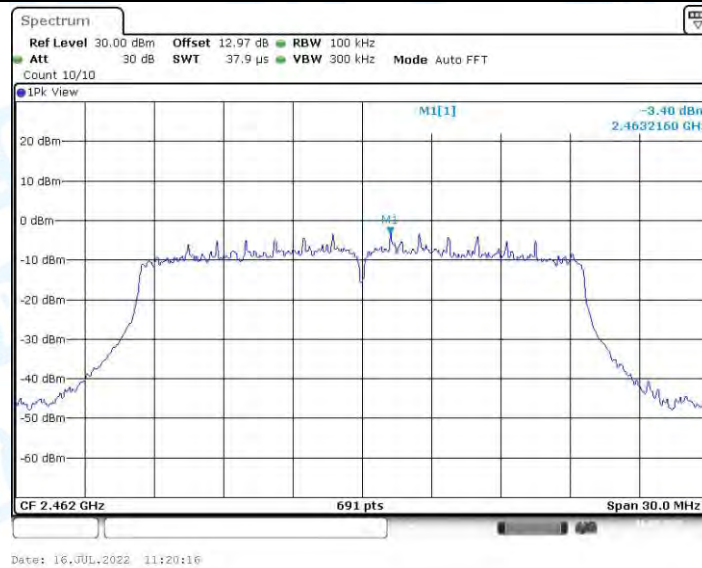
11AX20MIMO_Ant0_2462_0~Reference
