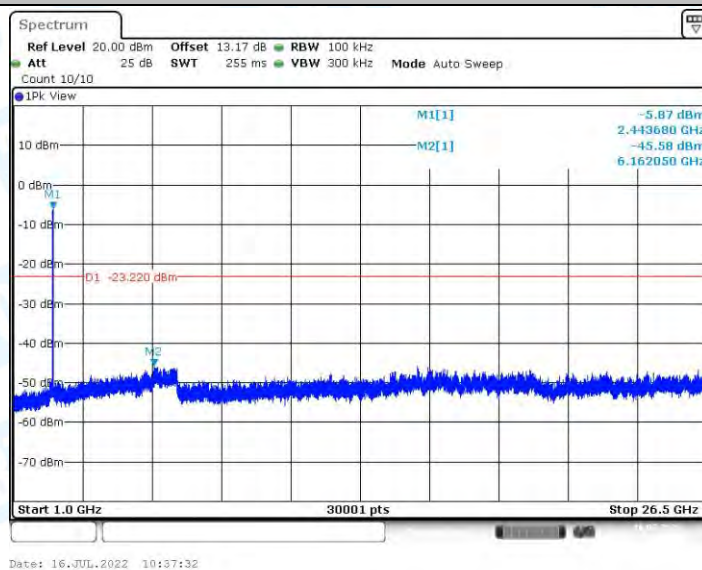
11N20MIMO_Ant1_2437_1000~26500
