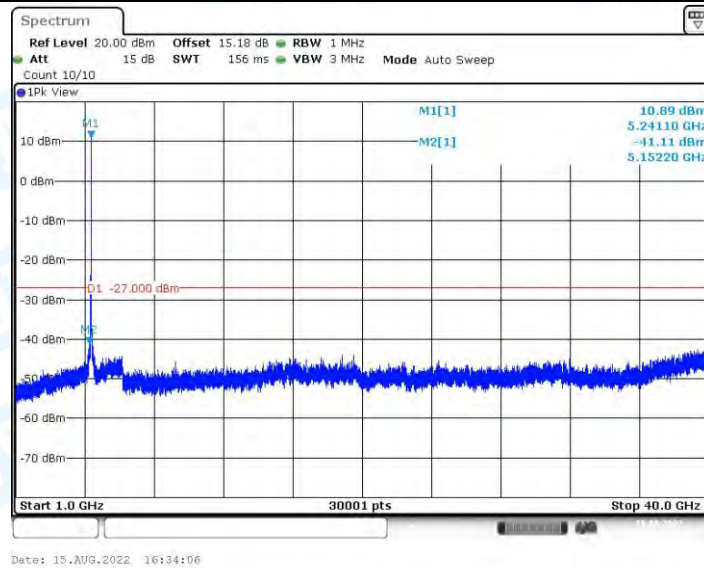
11AX20MIMO_Ant0_5240_1000~40000
