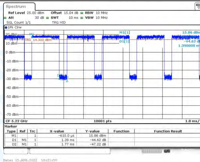
11A-CDD_Ant0_5220
