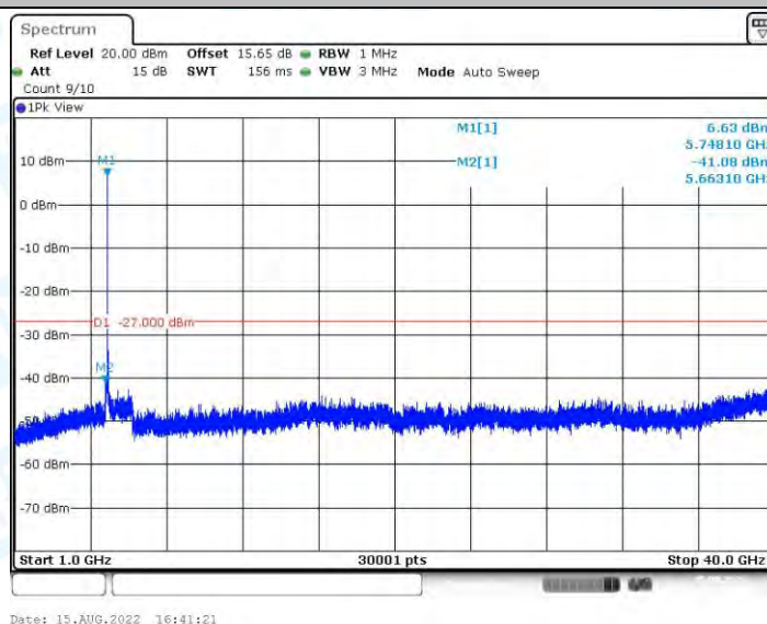
11AX20MIMO_Ant0_5745_1000~40000
