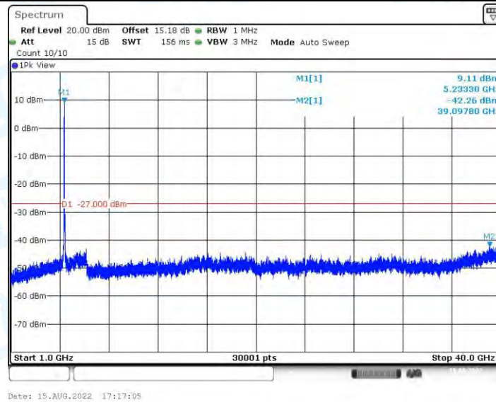
11AX40MIMO_Ant0_5230_1000~40000
