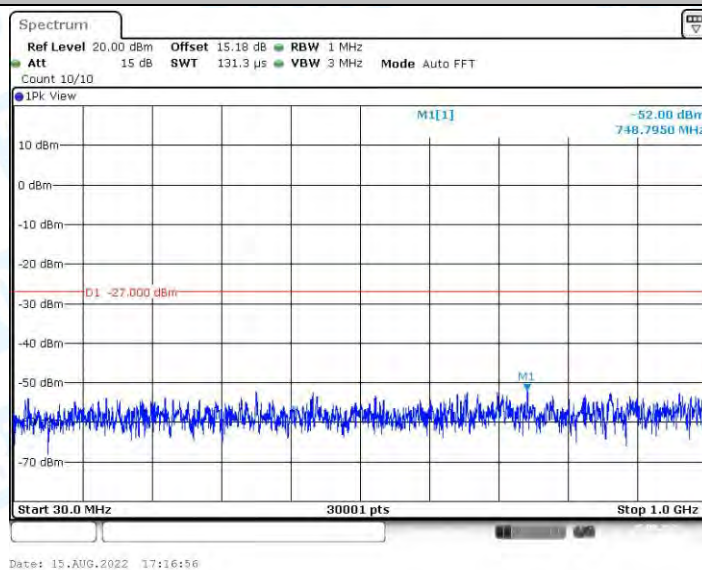
11AX40MIMO_Ant0_5230_30~1000
