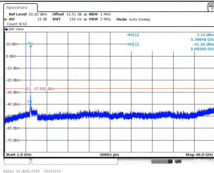
11AX20MIMO_Ant1_5785_1000~40000
