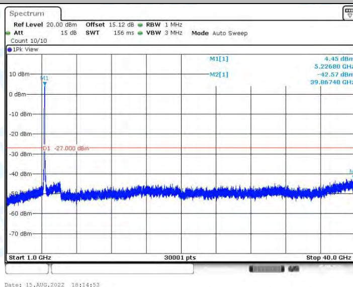
11AX80MIMO_Ant1_5210_1000~40000
