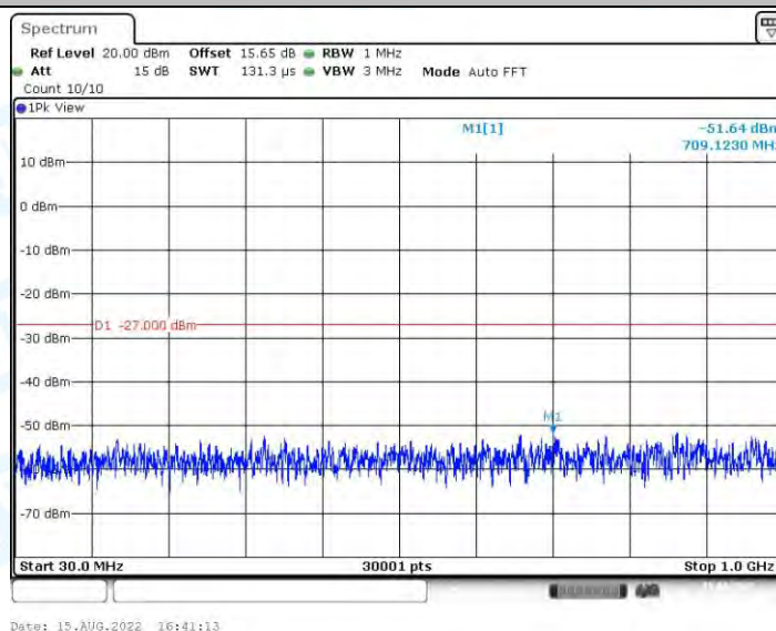
11AX20MIMO_Ant0_5745_30~1000
