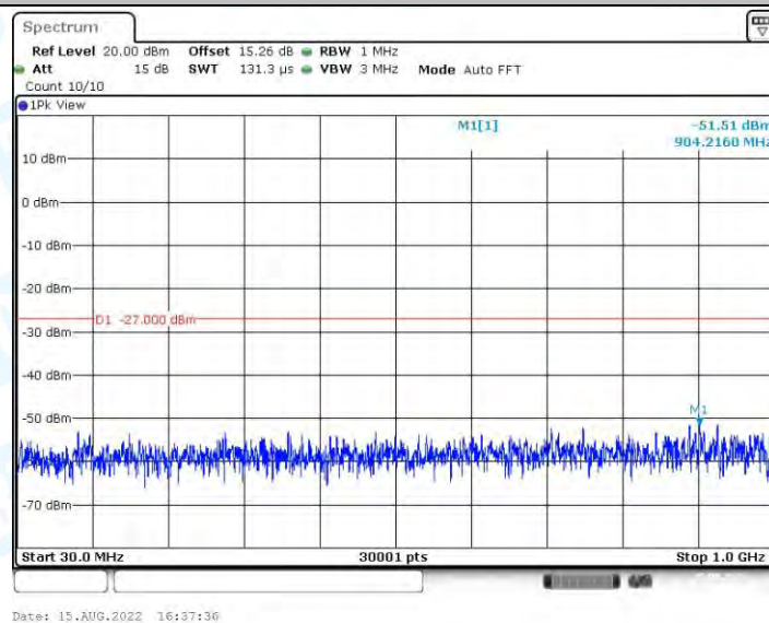
11AX20MIMO_Ant1_5240_30~1000
