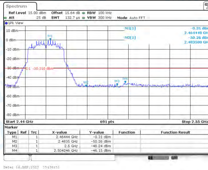
11AX20MIMO_Ant2_High_2462
