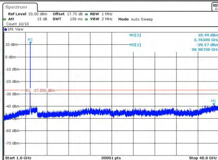
11N40MIMO_Ant2_5755_1000~40000
