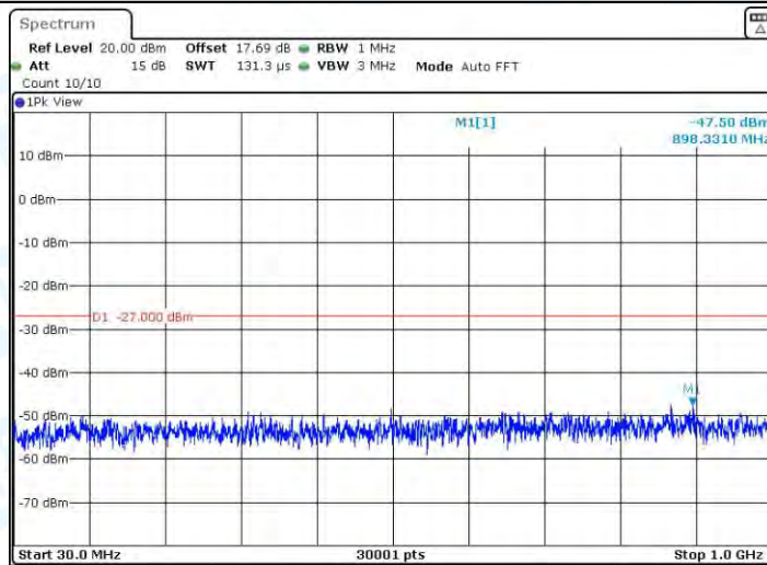
11N40MIMO_Ant1_5795_30~1000
