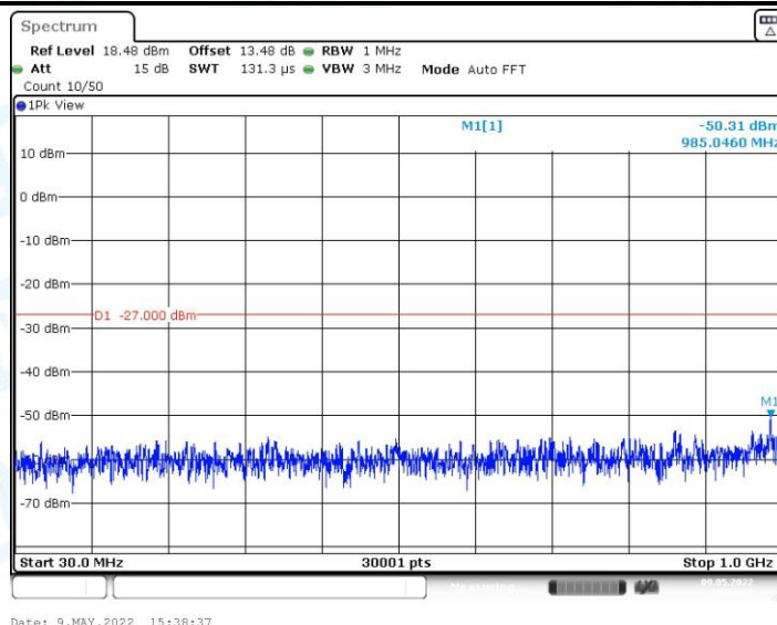
11N40MIMO_Ant0_5190_30~1000
