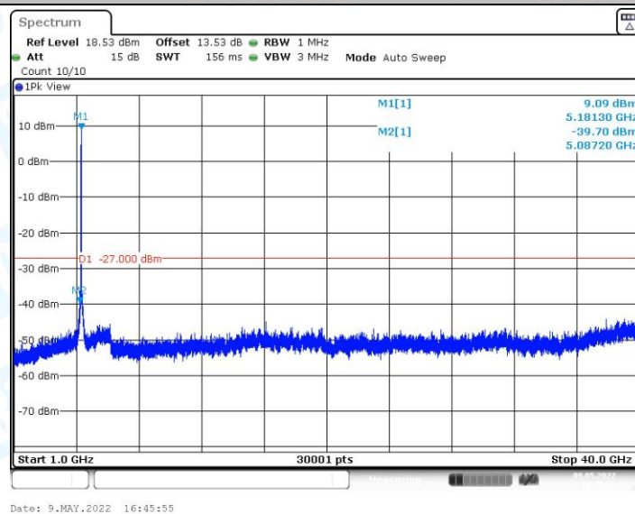
11AC20MIMO_Ant0_5180_1000~40000
