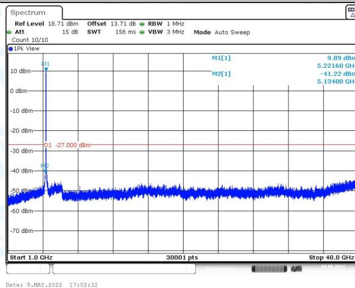
11AC20MIMO_Ant1_5220_1000~40000
