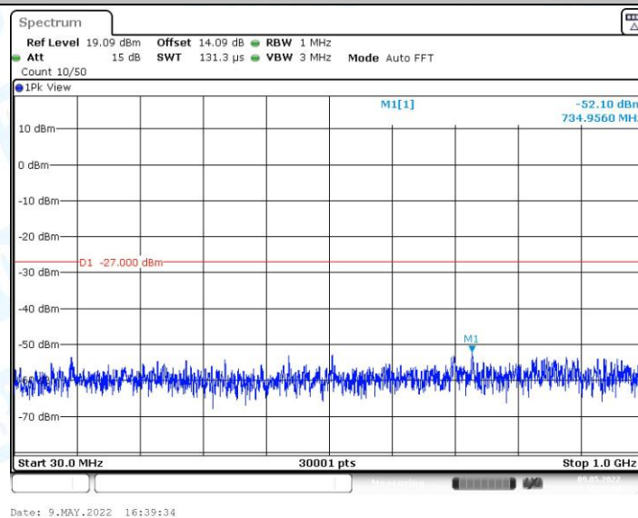
11N40MIMO_Ant1_5795_30~1000
