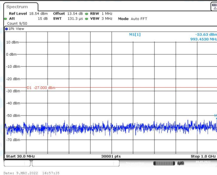
11AC20MIMO_Ant0_5220_30~1000
