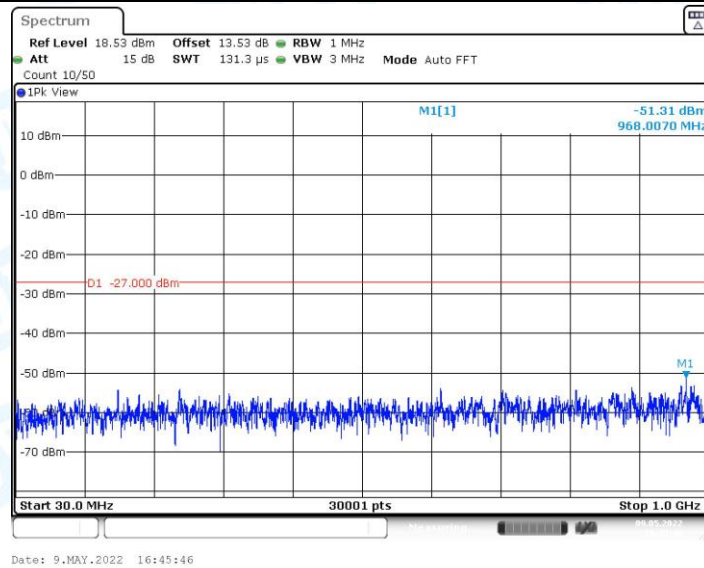
11AC20MIMO_Ant0_5180_30~1000
