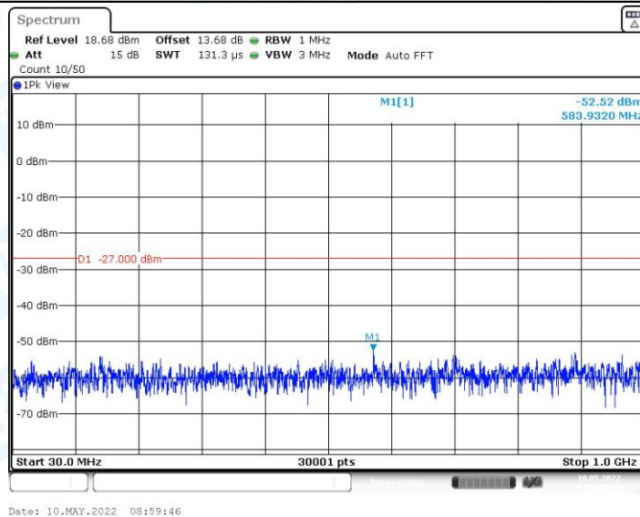
11AC40MIMO_Ant0_5230_30~1000
