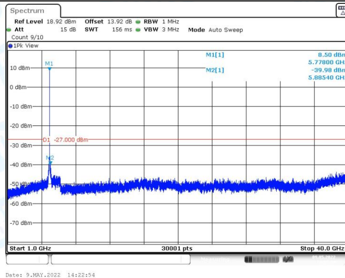
11N20MIMO_Ant0_5785_1000~40000
