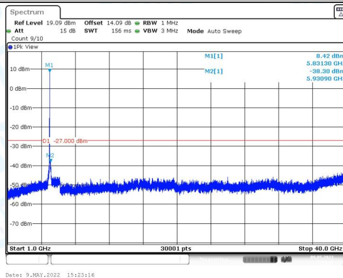
11N20MIMO_Ant1_5825_1000~40000
