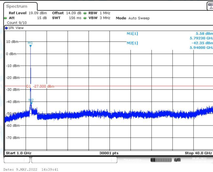
11N40MIMO_Ant1_5795_1000~40000
