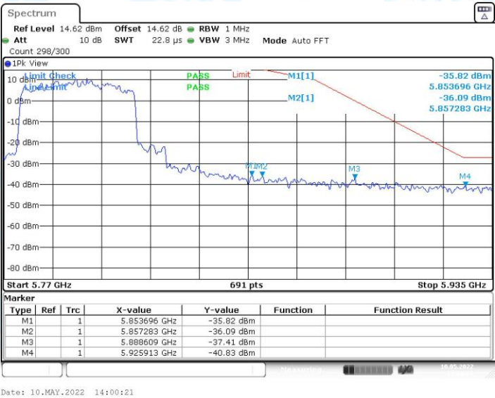
11AX40MIMO_Ant0_High_5795
