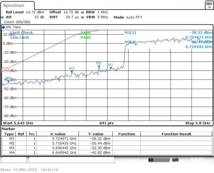
11AX80MIMO_Ant0_Low_5775
