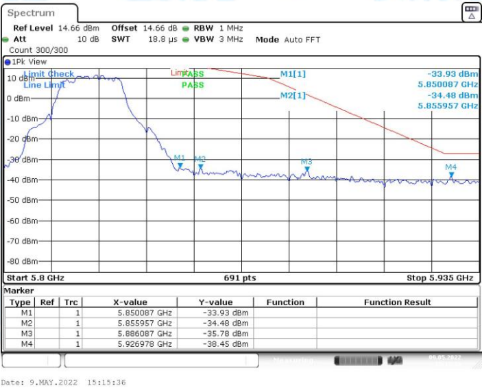
11N20MIMO_Ant0_High_5825
