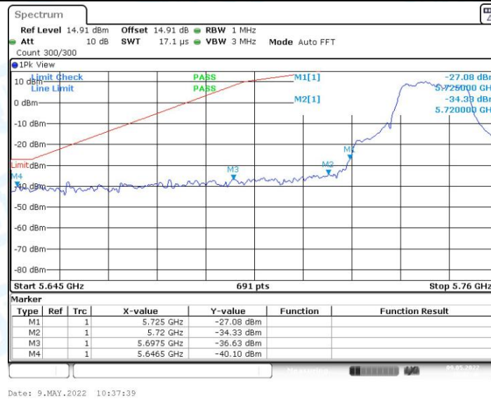
11AMIMO_Ant1_Low_5745
