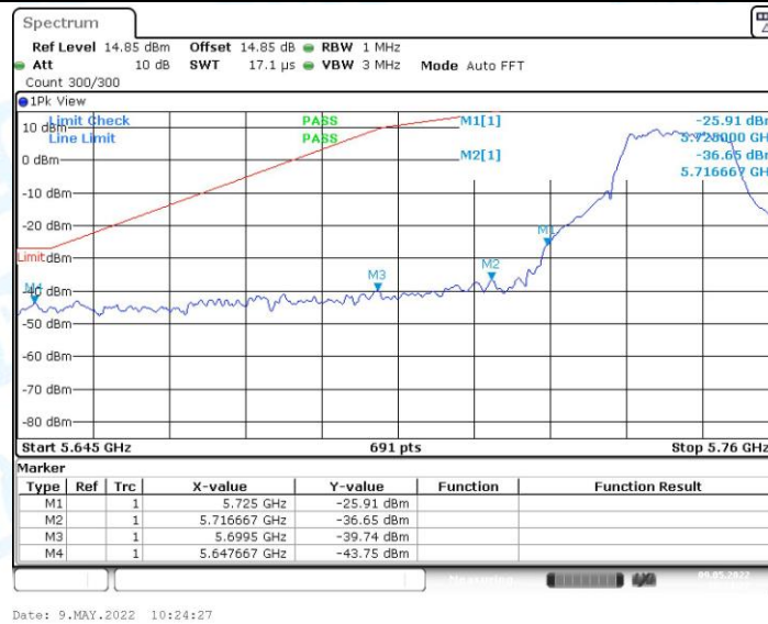
11AMIMO_Ant0_Low_5745
