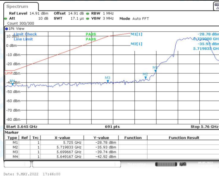
11AC20MIMO_Ant1_Low_5745
