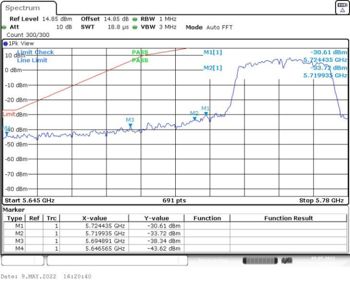
11N40MIMO_Ant0_Low_5755
