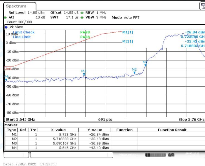
11AC20MIMO_Ant0_Low_5745
