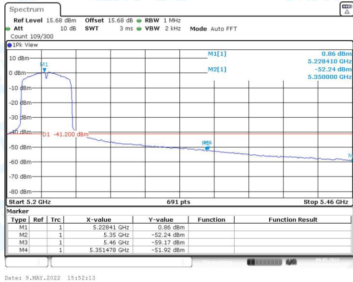
11N40MIMO_Ant0_High_5230_AV
