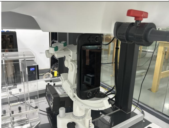
Left(dist. 0mm)
