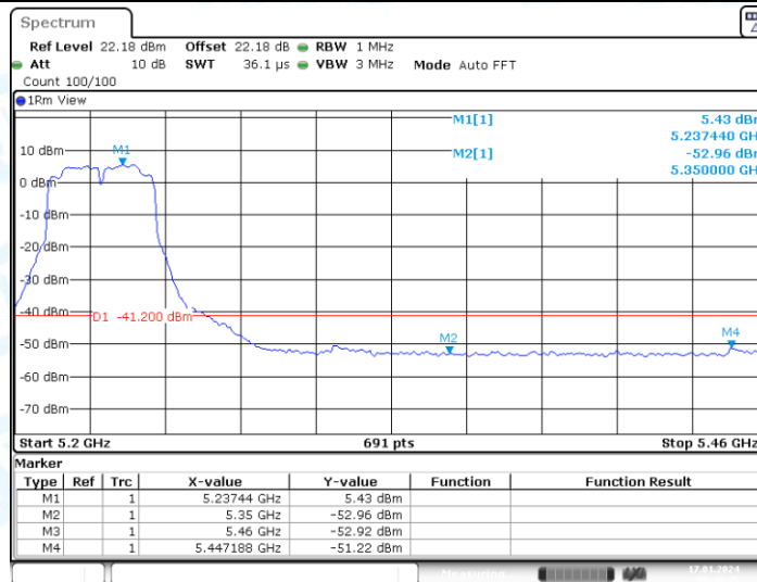
11N40MIMO_Ant2_High_5230_AV
